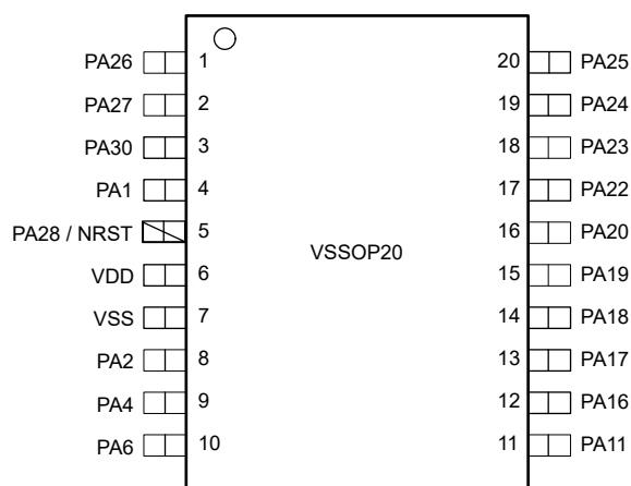
图 6-6. 20 引脚 DGS20 (VSSOP) (顶视图)
