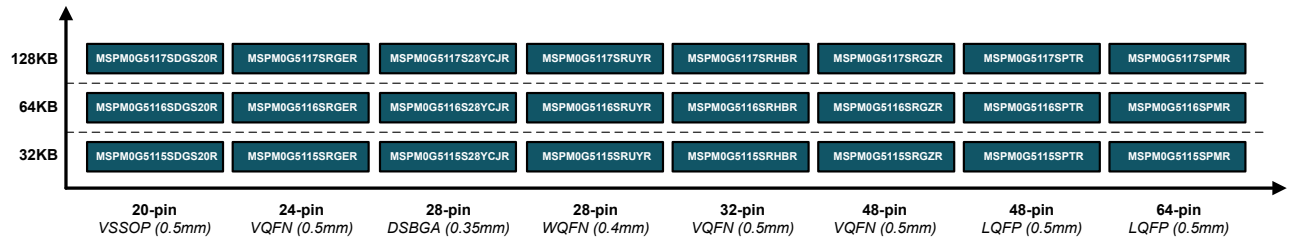
图 5-1. 器件比较图
