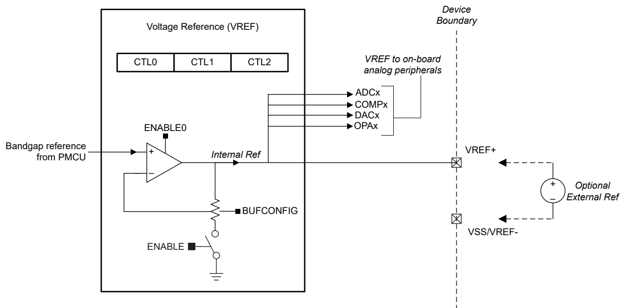
图 8-1. VREF 模块
