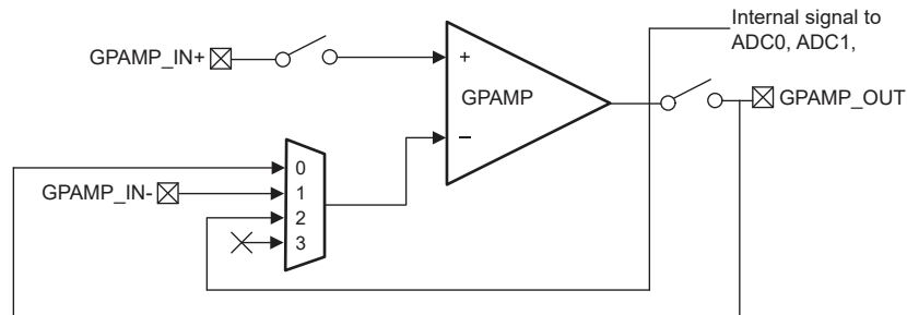
图 8-2. 模拟连接
