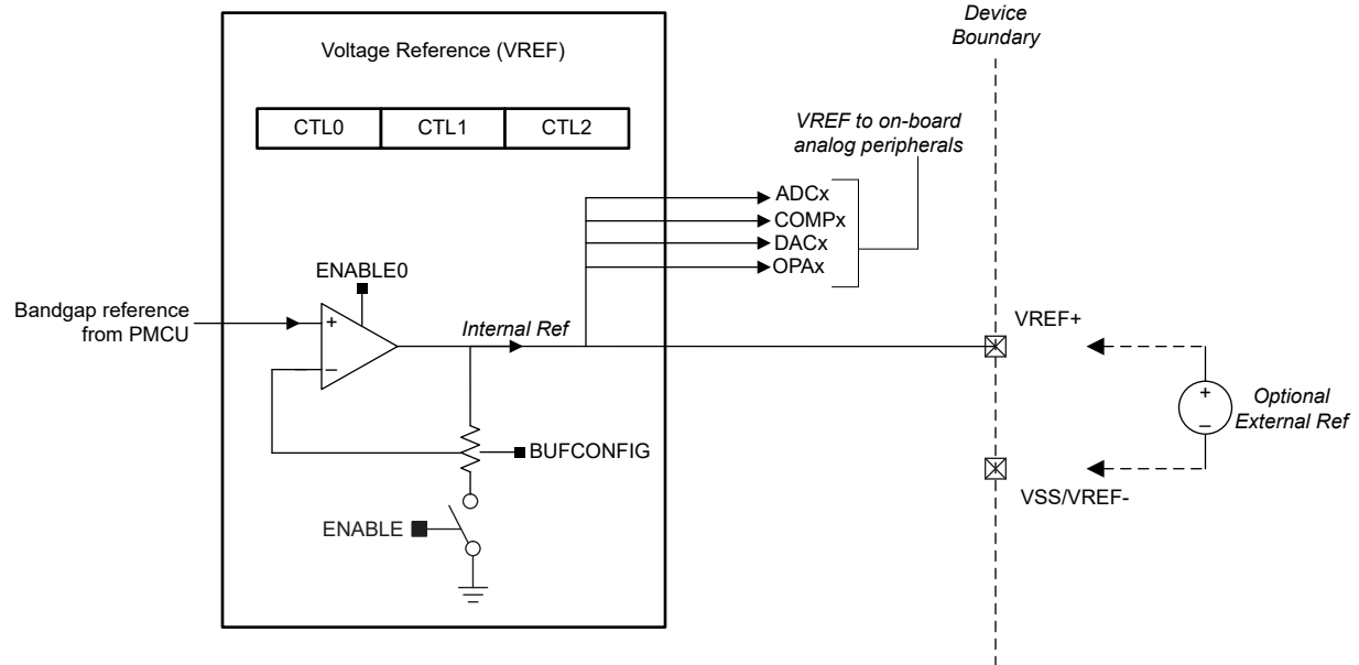
图 8-1. VREF 模块
