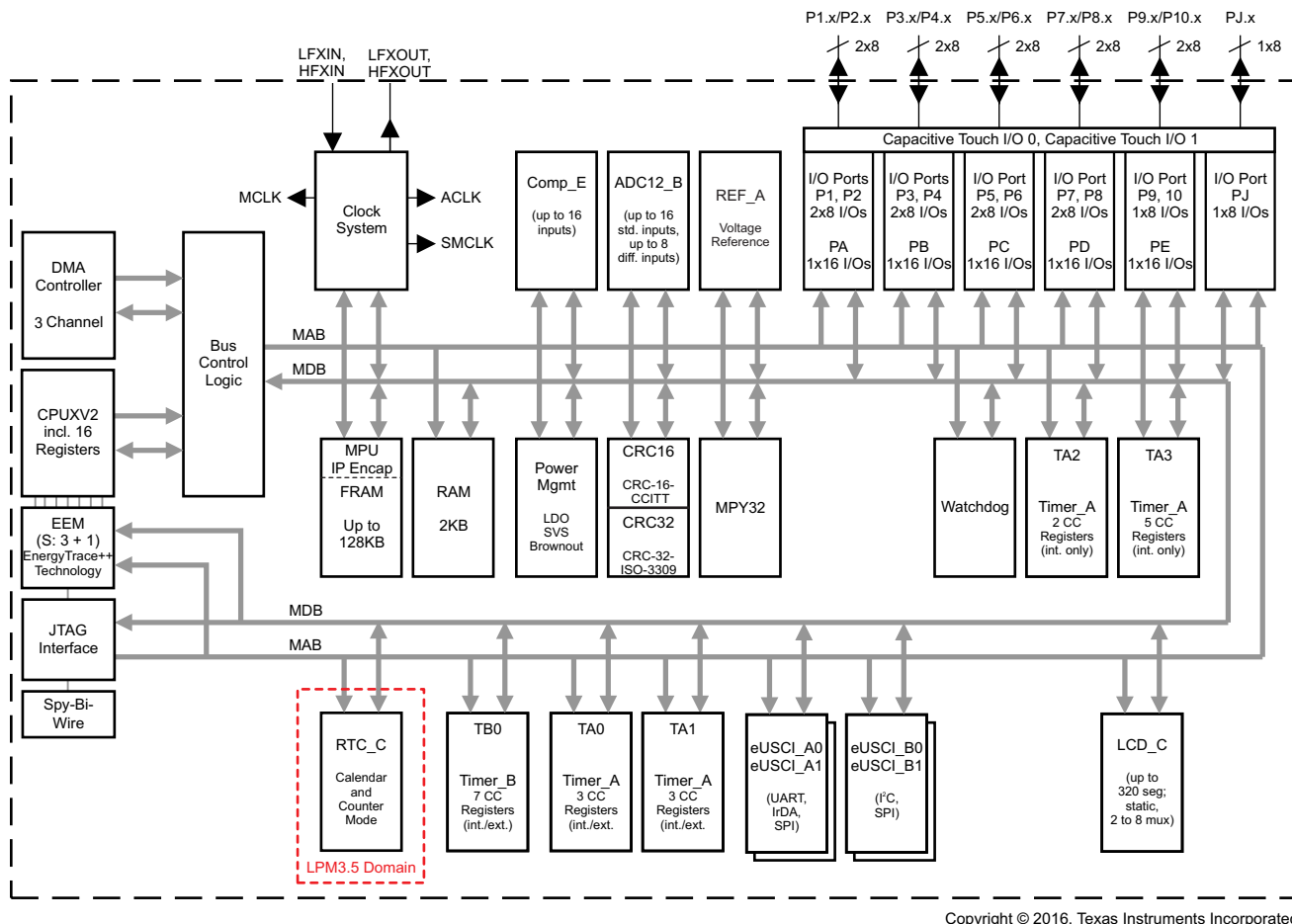
图 1-1. 功能方框图 – MSP430FR687x、MSP430FR687x1
