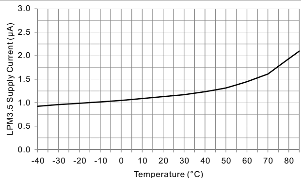
图 8-2. LPM3.5 电源电流与温度间的关系
