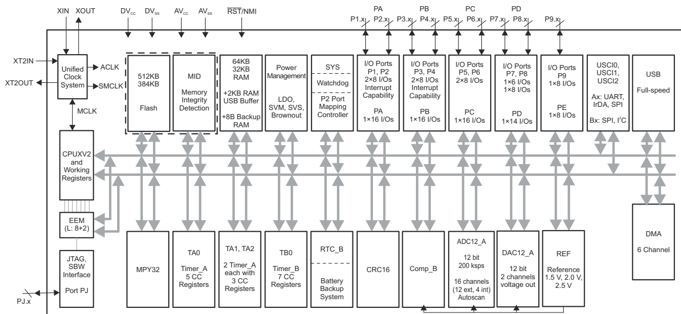
图 4-2. 功能方框图 - MSP430F5659、MSP430F5658
