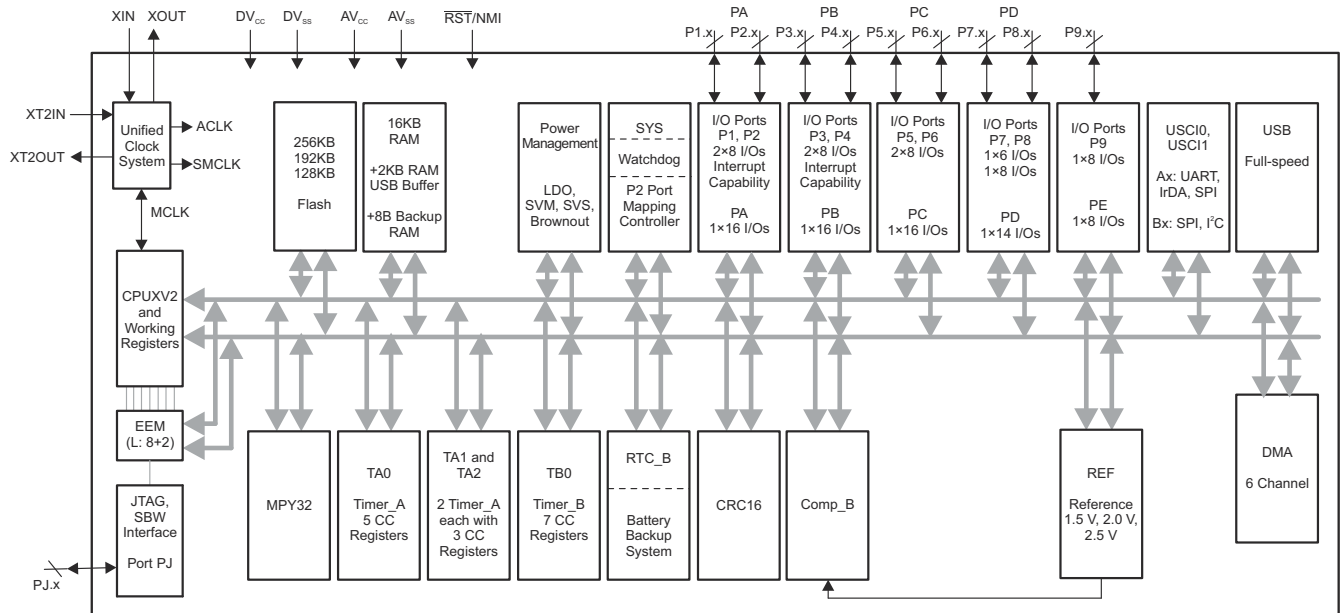
图 4-3. 功能框图 - MSP430F5632、MSP430F5631 和 MSP430F5630
