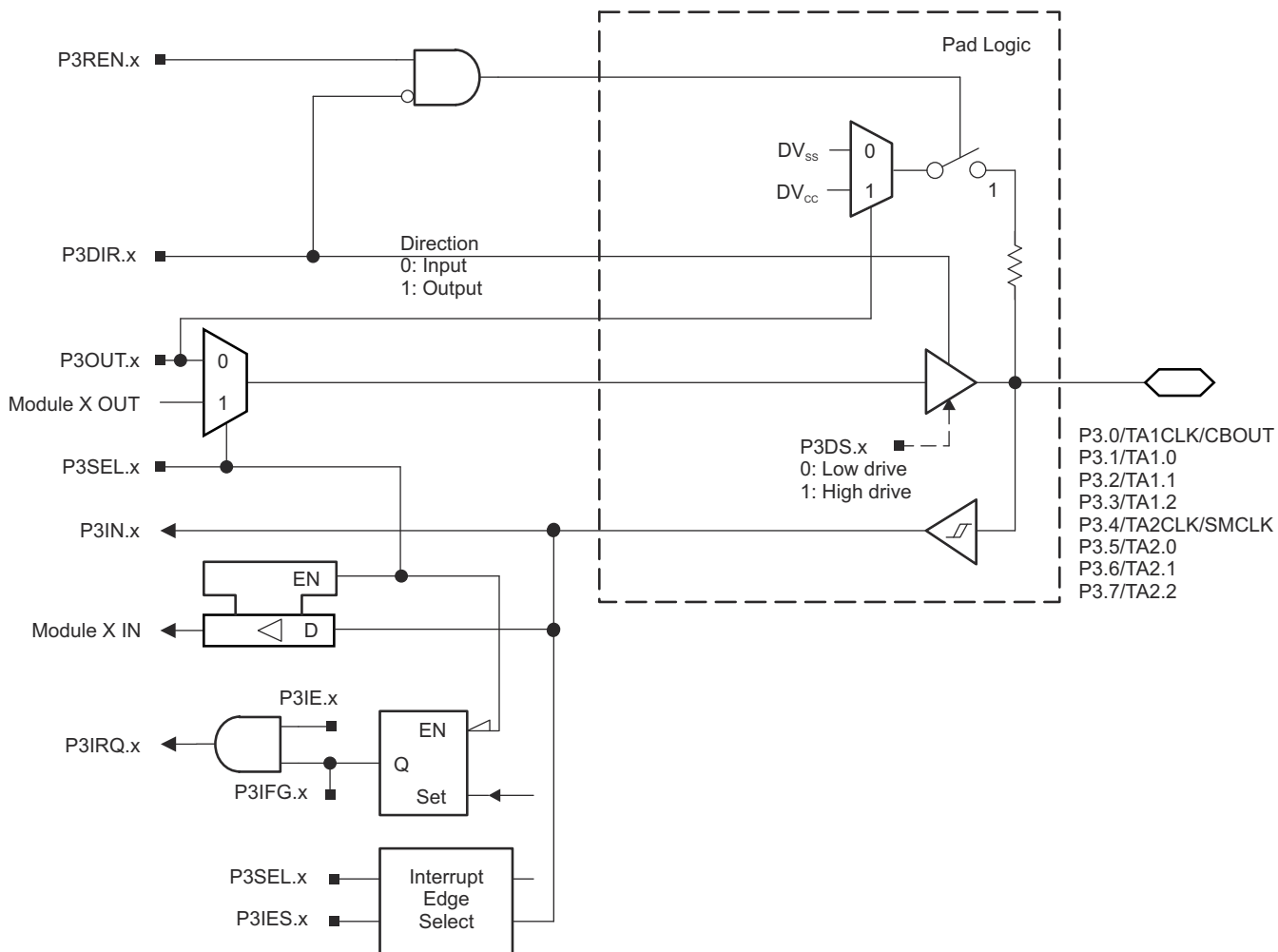
图 9-4. Port P3 (P3.0 to P3.7) Diagram
