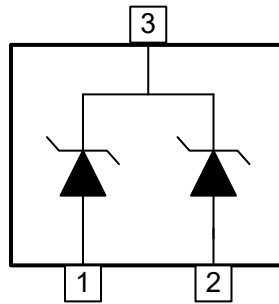
功能图
