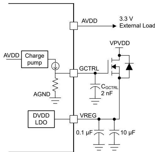
图 7-6. 用于 VREG 的外部 MOSFET 稳压器
