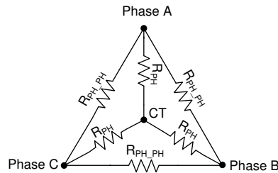
图 7-38. 电机电阻
