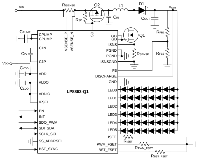
简化原理图
