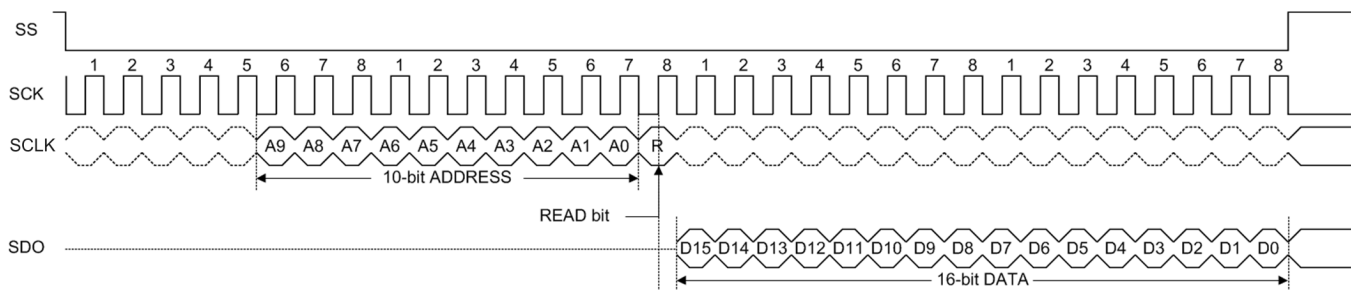
图 31. SPI Read
