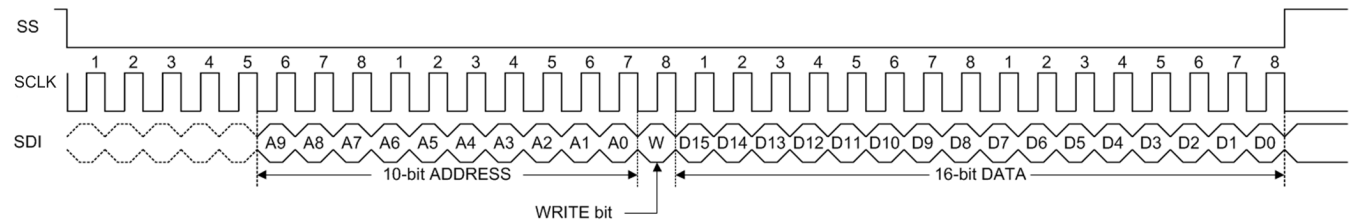
图 30. SPI Write
