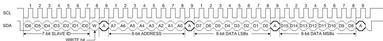
图 32. I2C Write
