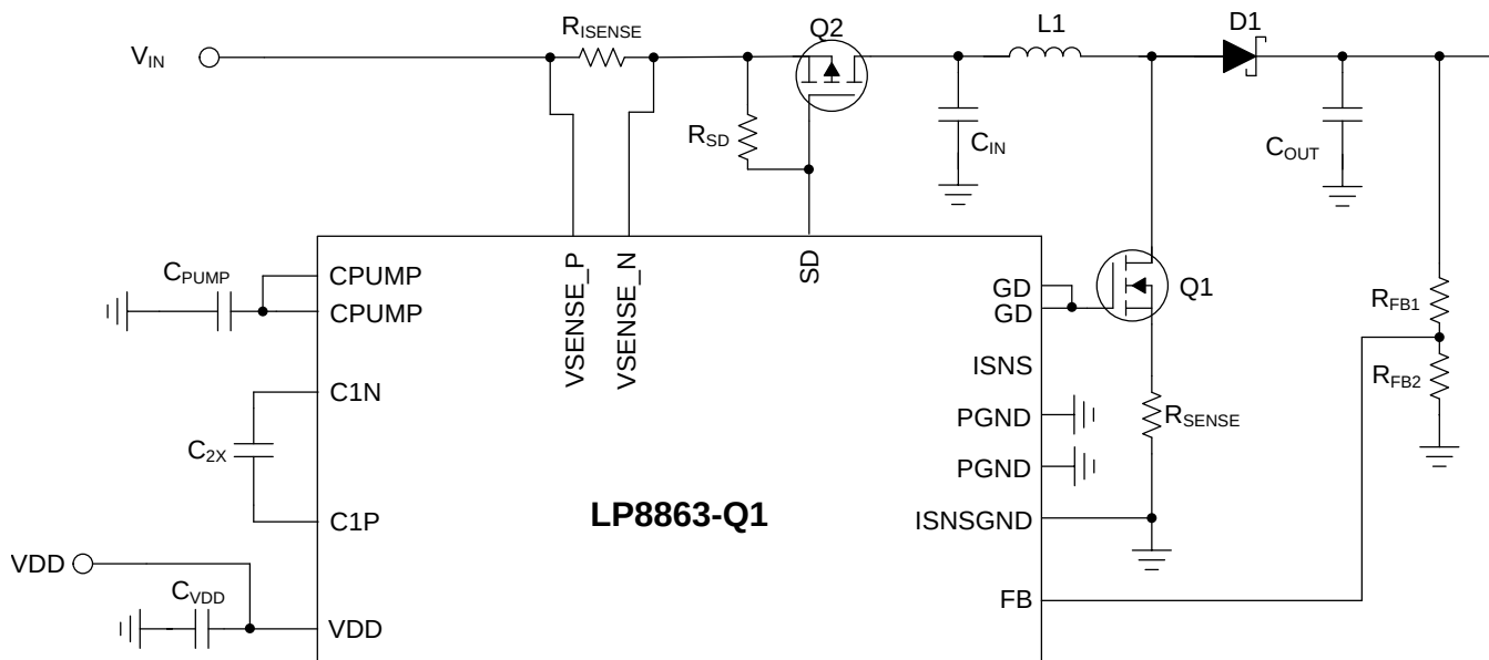
图 14. Charge Pump Enabled Circuit
