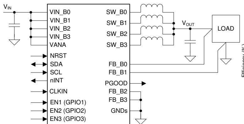
简化原理图
