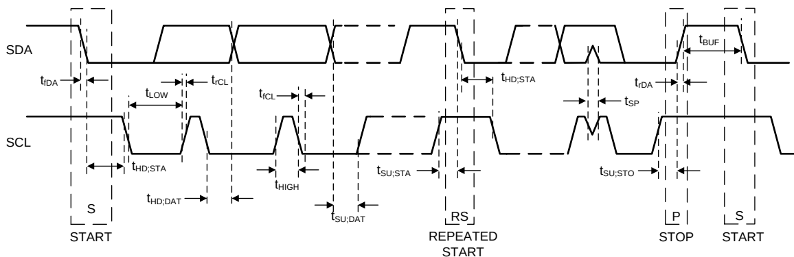
图 24. I²C-Compatible Timing
