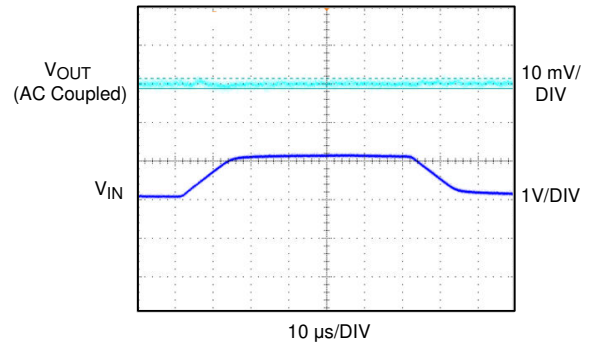
图 5-8. 线路调整
