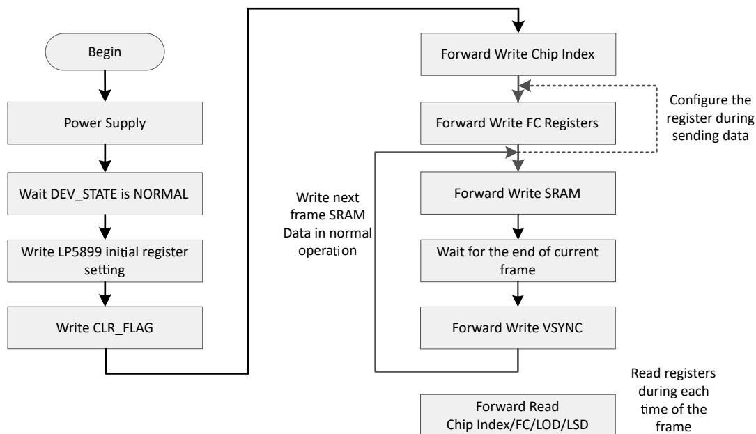
图 8-2. 编程过程
