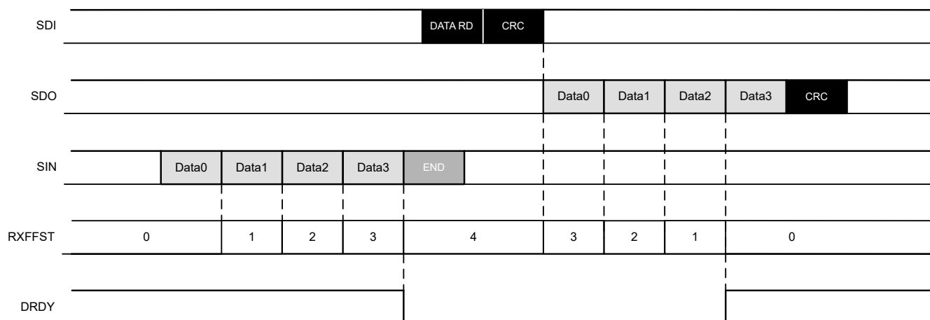
图 7-7. RXFFLVL 寄存器设置为 3 时的 DRDY 引脚示例
