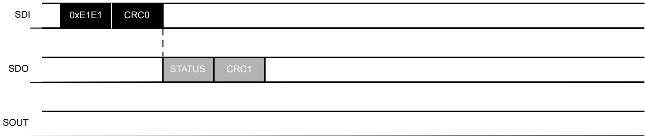
图 7-21. SOFTRESET_CRC 命令示例
