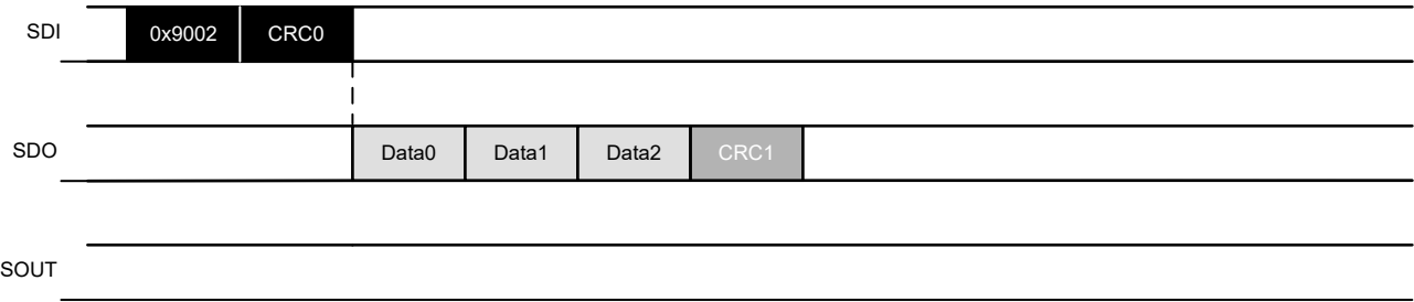
图 7-16. DATA_RD 命令示例
