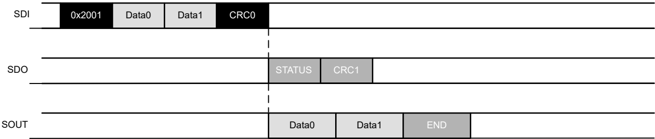
图 7-9. FWD_WR_CRC 命令示例
