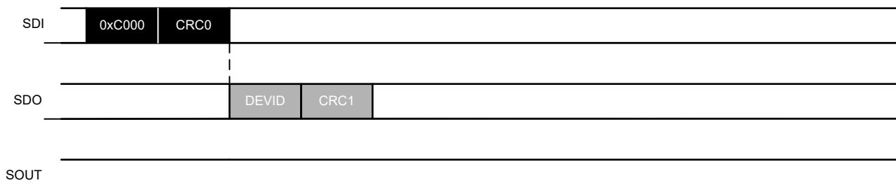
图 7-19. REG_RD_CRC 命令示例
