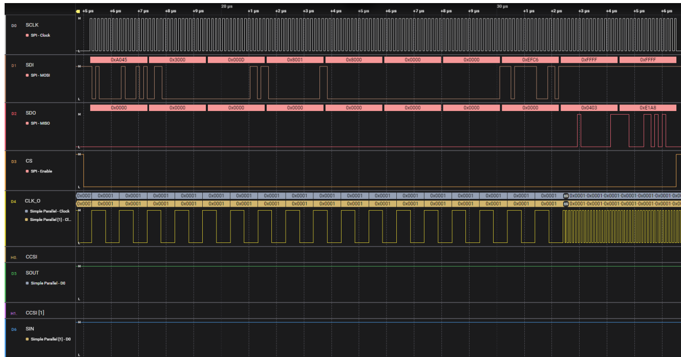
图 9-3. 写入初始寄存器设置示例
