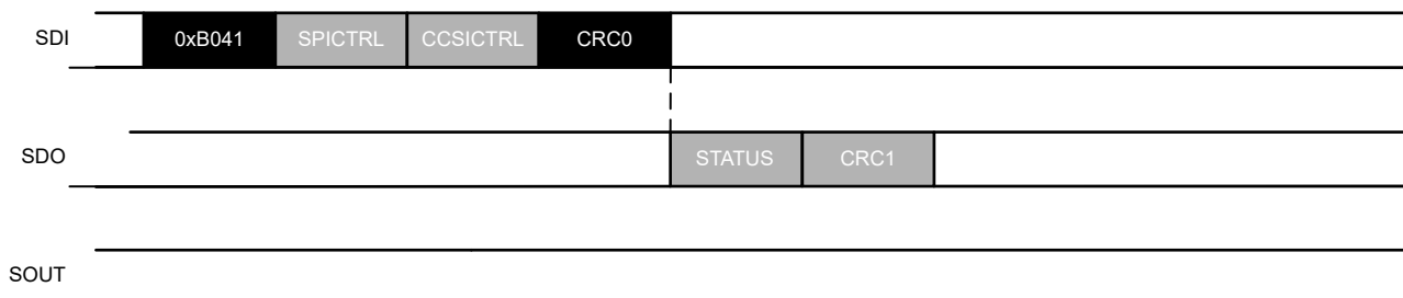
图 7-18. REG_WR 命令示例
