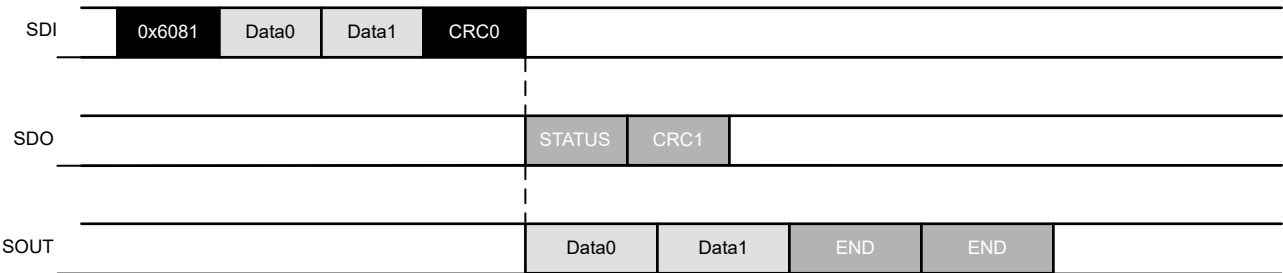
图 7-13. FWD_RD_END_CRC 命令示例
