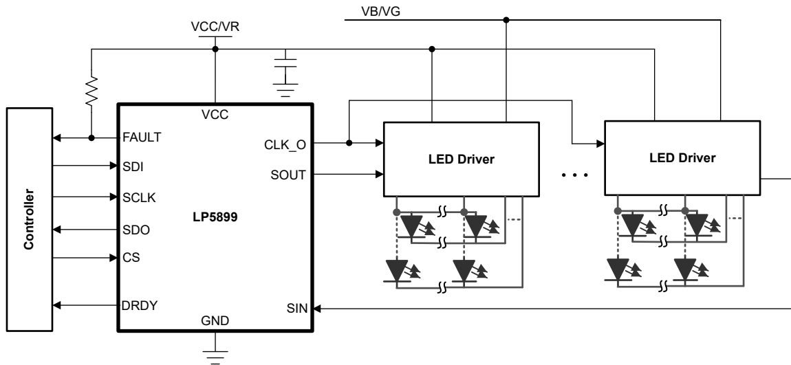
典型应用图
