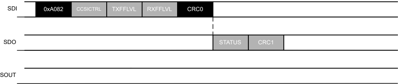
图 7-17. REG_WR_CRC 命令示例
