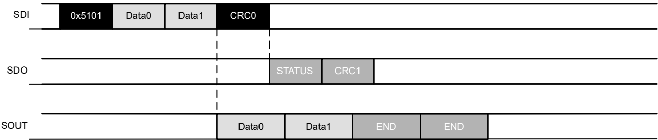
图 7-12. FWD_WR_END 命令示例
