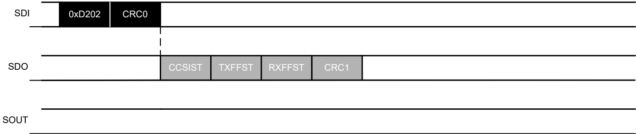
图 7-20. REG_RD 命令示例
