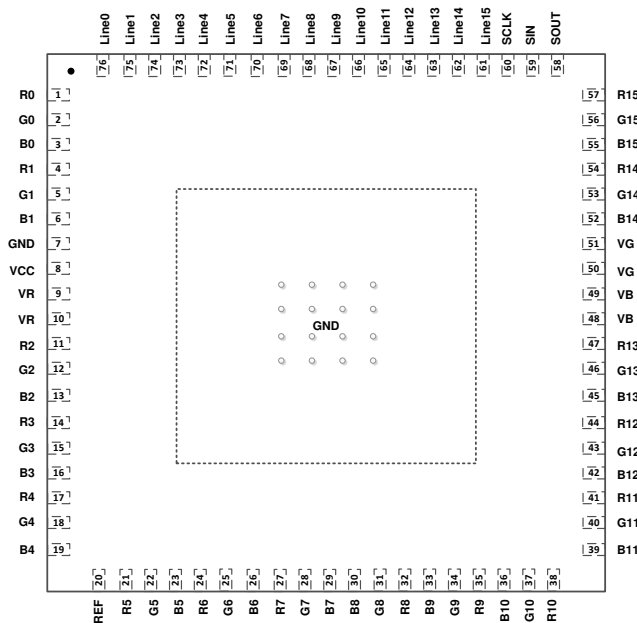
图 4-1. LP5892-Q1 RRF 封装 76 引脚 VQFN (带有外露散热焊盘) (顶视图)
