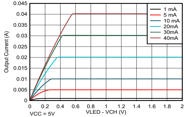
图 5-3. 通道电流与 (VLED-Vchannel) 电压间的关系
