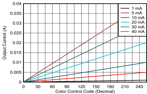
图 5-6. 颜色控制代码与输出电流间的关系
