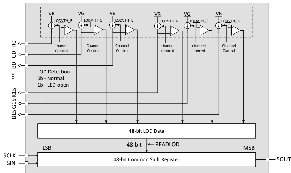
图 6-5. LED 开路检测电路
