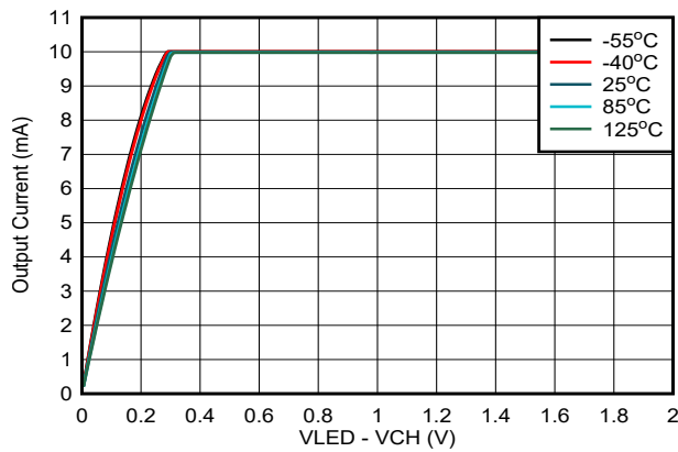
图 5-4. 通道电流与 (VLED-Vchannel) 电压间的关系
