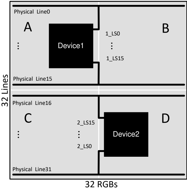
图 6-2. Mode2 示意图
