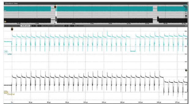
图 7-8. 单帧中的线路和通道波形 (GSn = 0x0001h)
