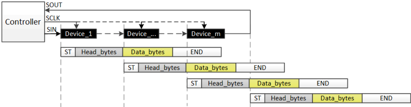
图 6-18. 使用广播的数据写入命令
