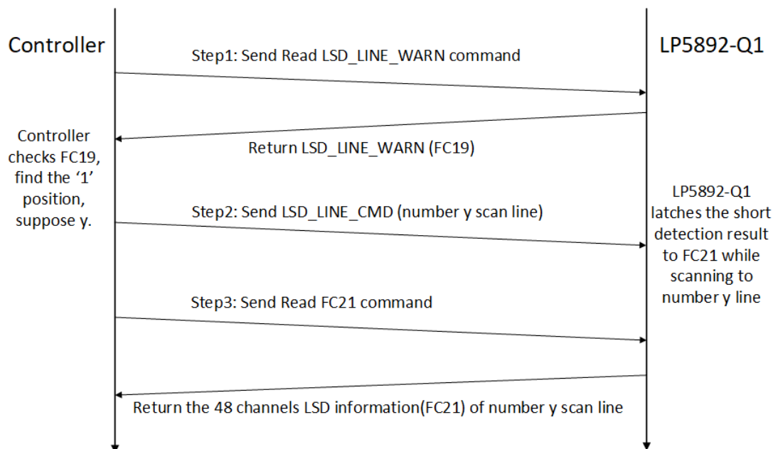
图 6-11. 读取 LED 短路信息的步骤
