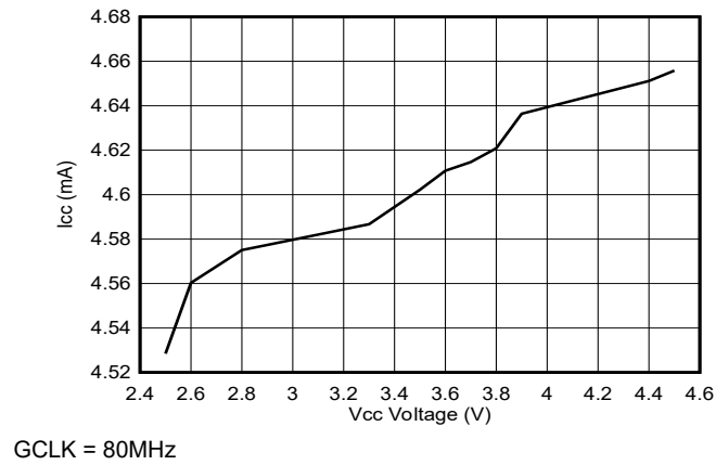
图 5-8. Icc 电流与 Vcc 电压间的关系
