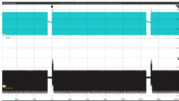
图 7-7. 单帧中的线路和通道波形 (GSn = 0x0001h)
