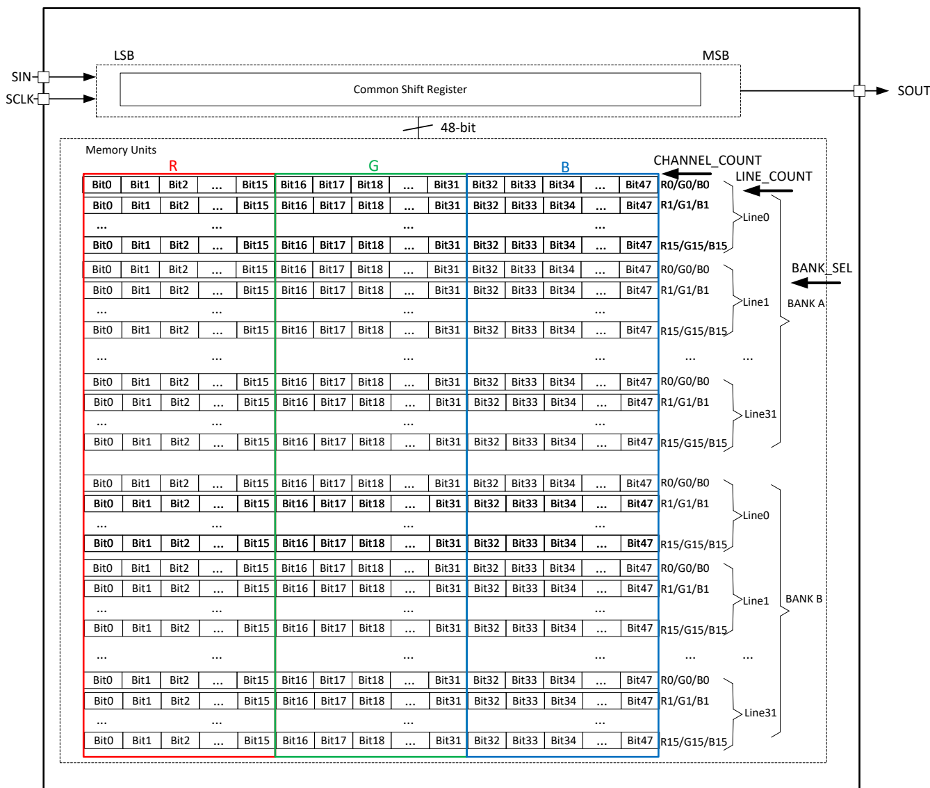
图 6-24. LP5892-Q1 存储器单元结构
