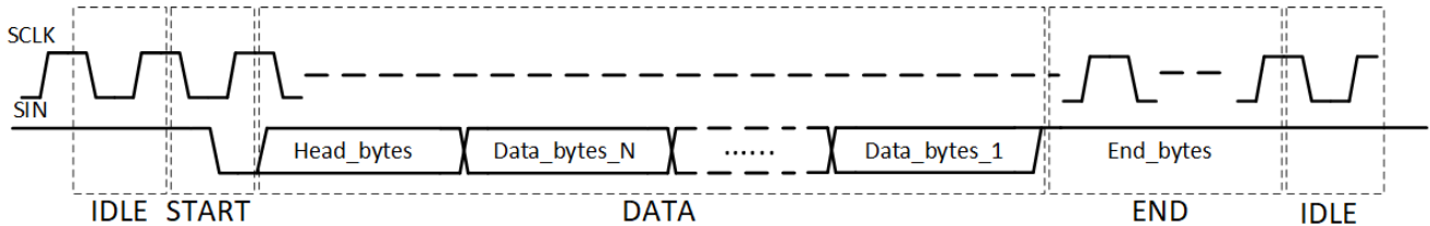
图 6-14. CCSI 帧
