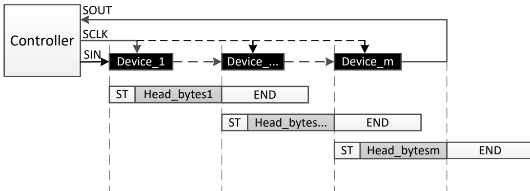
图 6-15. 芯片索引写入命令
