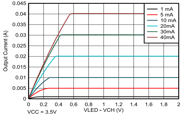
图 5-2. 通道电流与 (VLED-Vchannel) 电压间的关系
