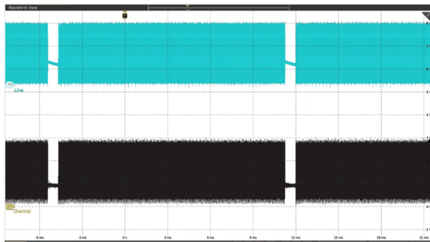
图 7-5. 单帧中的线路和通道波形 (GSn = 0xFFFFh)
