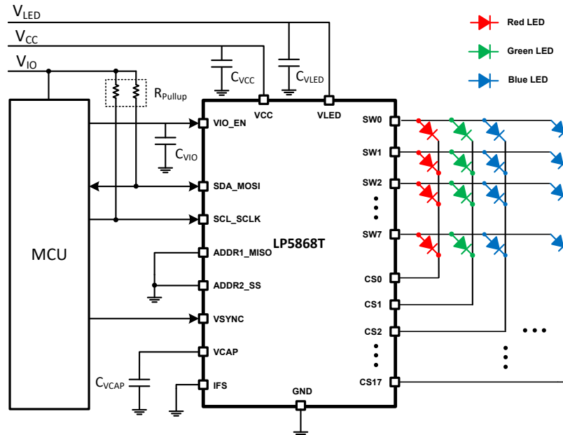
图 8-1. 典型应用 — LP5868T 驱动 48 个 RGB LED (144 个 LED 点阵)
