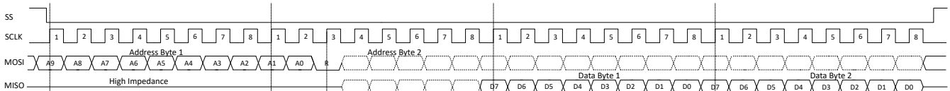
图 7-18. SPI 读取时序
