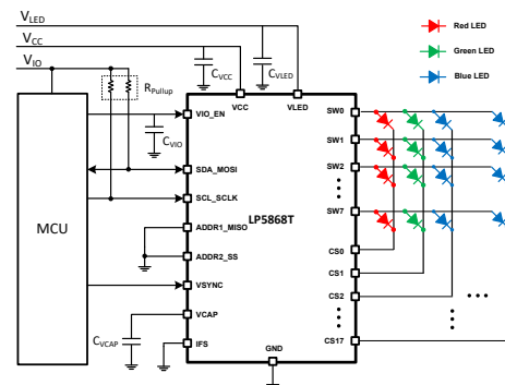
简化原理图
