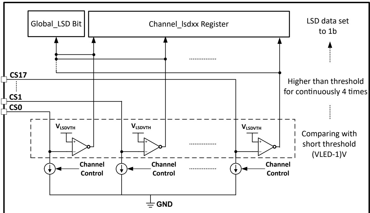
图 7-12. LSD 电路
