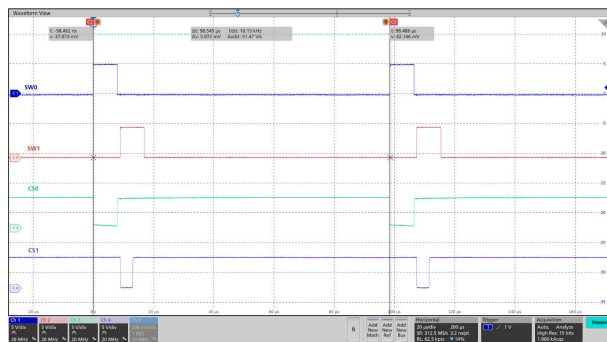
图 8-3. SW0、SW1、CS0、CS1 的扫描线和电流阱波形
