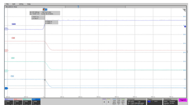
图 8-8. 已禁用 PWM 相移
