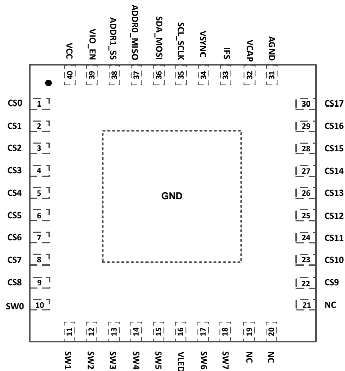
图 5-1. LP5868T RKP 封装 40 引脚 VQFN (带外露散热焊盘) 顶视图
