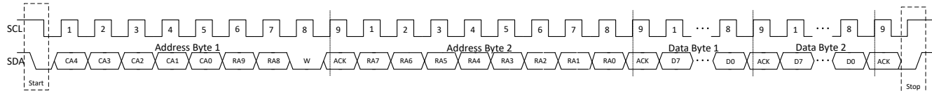
图 7-14. I²C Write Timing
