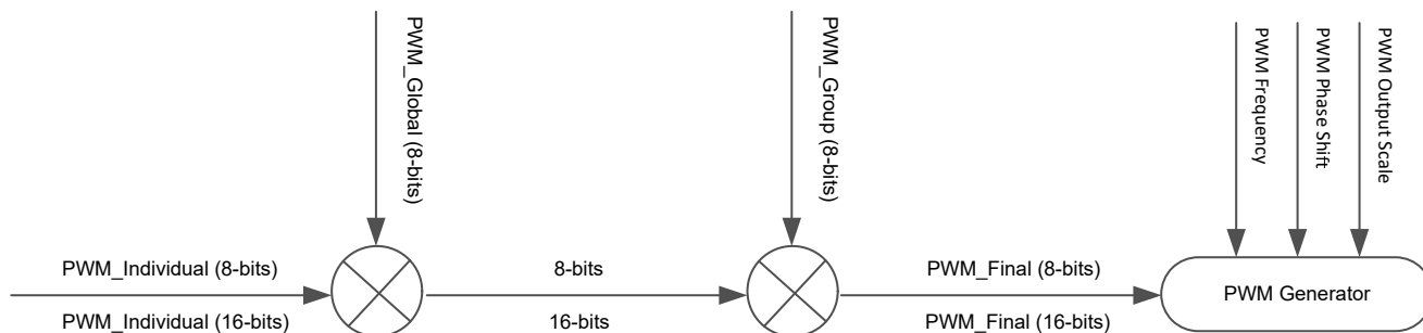
图 7-6. PWM Control Scheme
