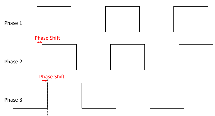
图 7-4. Phase Shift
