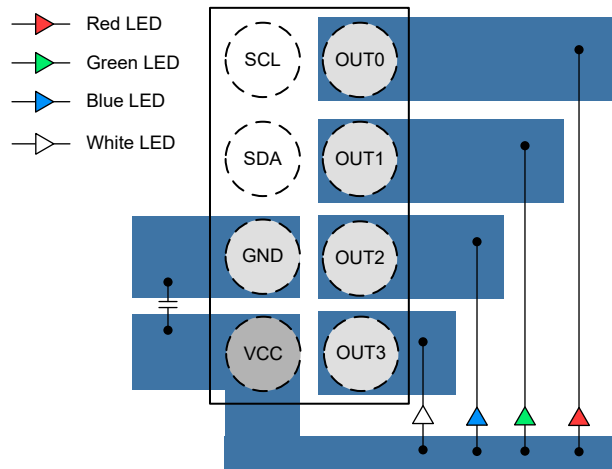
图 8-8. LP5814 YCH 封装布局示例
