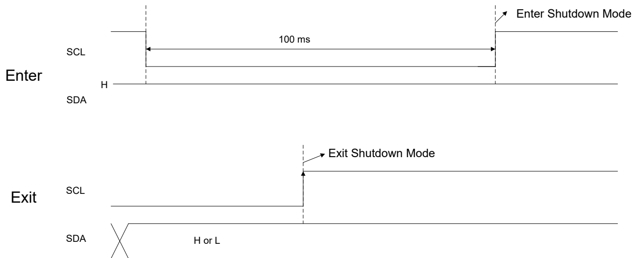
图 7-11. 进入和退出关断模式方法对 2
