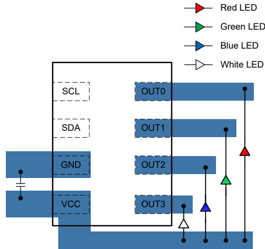
图 8-7. LP5814 DRL 封装布局示例
