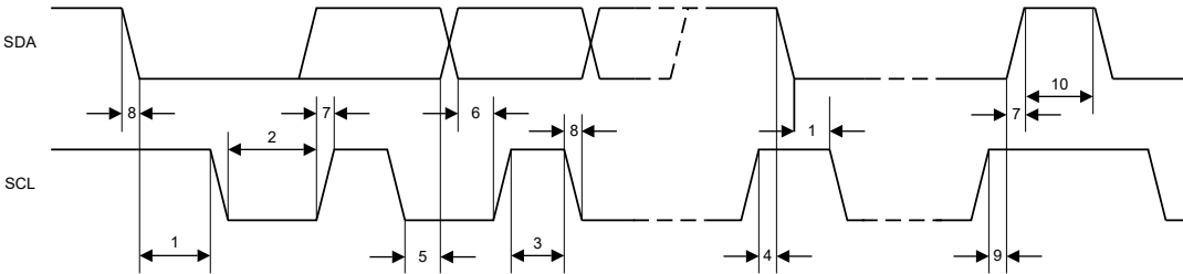
图 6-1. I 2 C 时序参数
