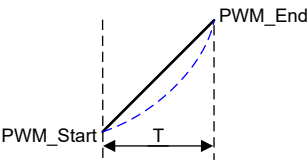
图 7-3. Sloper 曲线演示
