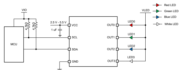
LP5814 简化原理图
