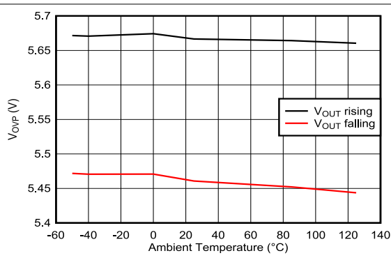
图 6-2. VOUT OVP 阈值
