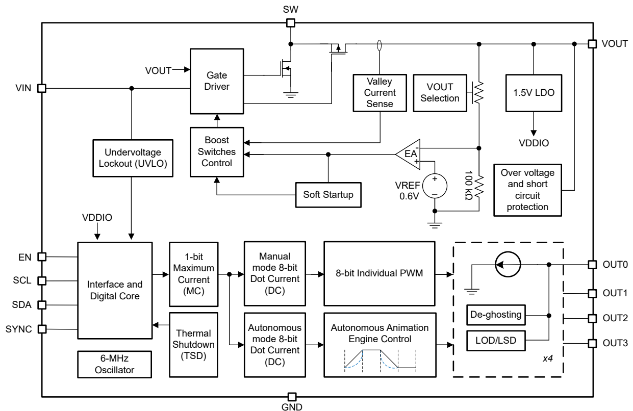
图 7-1. 功能方框图
