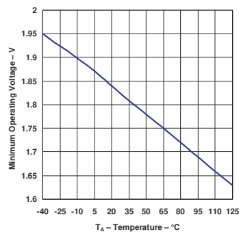
图 5-27. 最低工作电压与温度之间的关系 (旧芯片)
