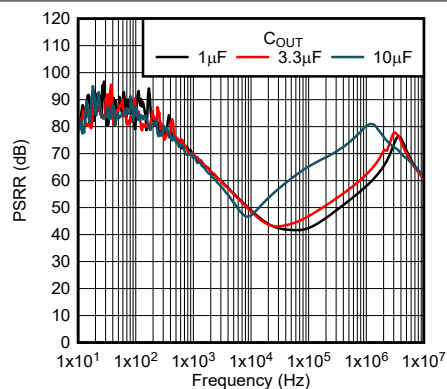
图 5-58. 纹波抑制与频率之间的关系 (新芯片)
