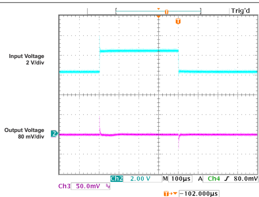
图 5-45. 线路瞬态响应与时间之间的关系 (旧芯片)
