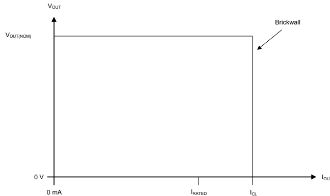
图 6-2. 电流限制
