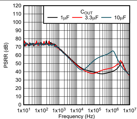
图 5-59. 纹波抑制与频率之间的关系 (新芯片)
