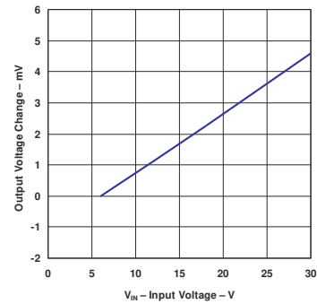
图 5-40. 线性调整率与输入电压之间的关系 (旧芯片)
