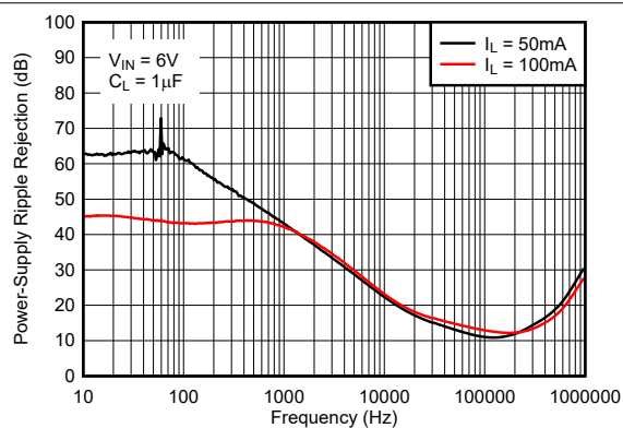
图 5-57. 纹波抑制与频率之间的关系 (旧芯片)
