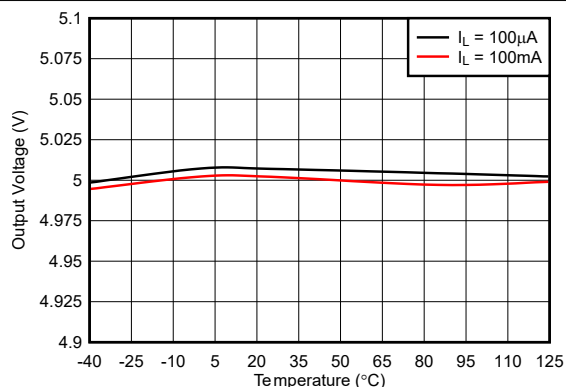
图 5-9. 输出电压与温度之间的关系 (旧芯片)
