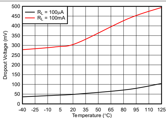
图 5-23. 压降电压与温度之间的关系 (旧芯片)
