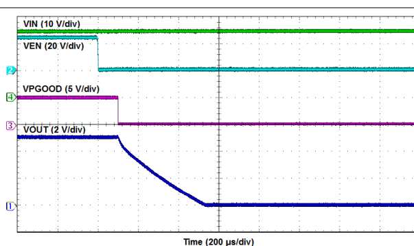
图 7-12. Enable Turn-OFF
