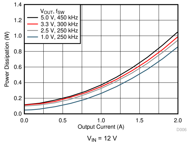
图 6-6. Power Dissipation vs Output Current
