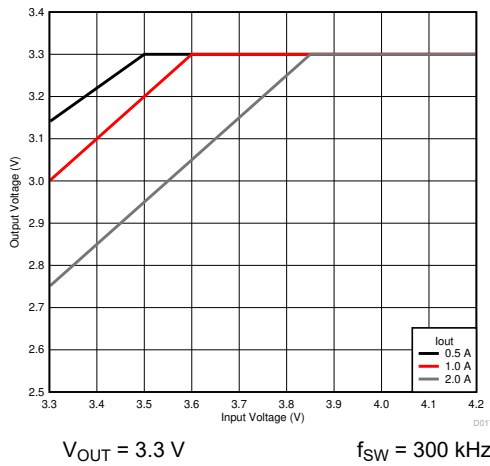
图 7-2. Voltage Dropout
