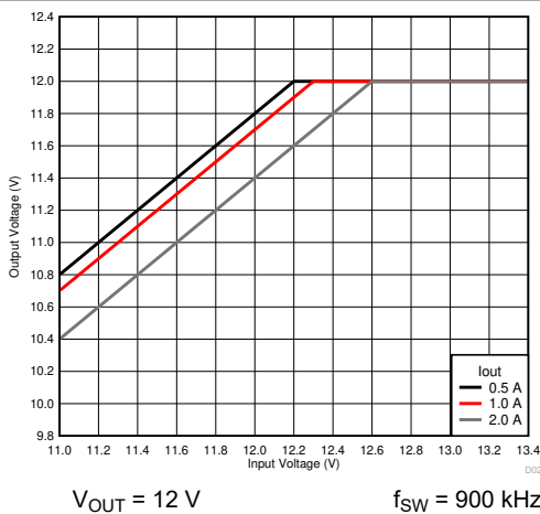
图 7-6. Voltage Dropout
