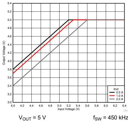
图 7-4. Voltage Dropout
