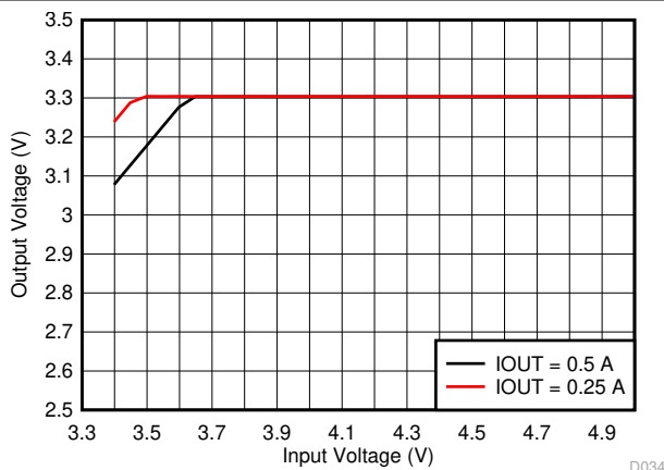
图 7-3. Dropout Voltage
