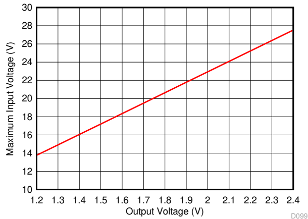
图 7-1. Maximum Input Voltage for V_{OUT} < 2.5\text{ V}
