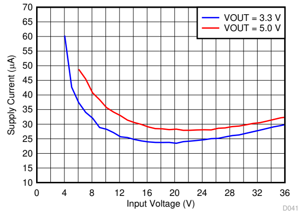
图 7-2. Input Supply Current
