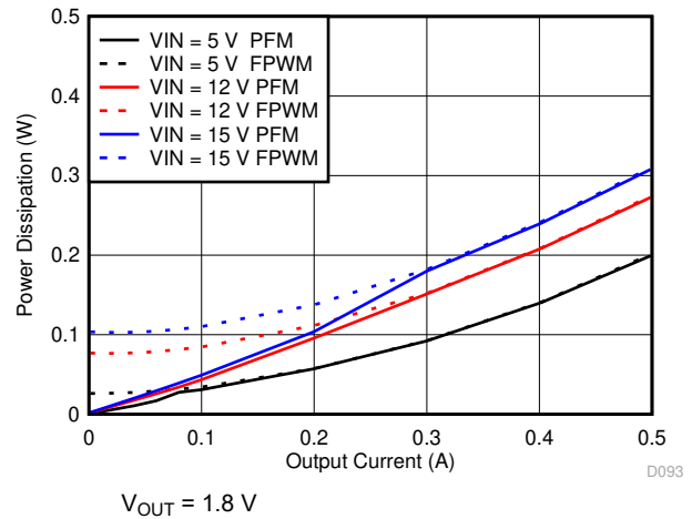
图 7-14. Power Dissipation
