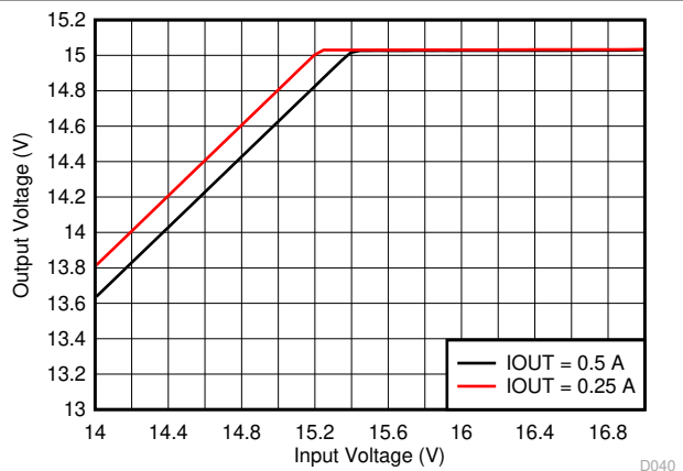
图 7-4. Dropout Voltage
