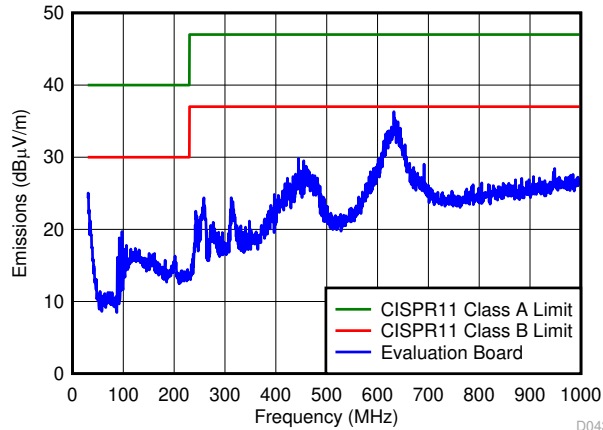
图 7-7. Radiated EMI
