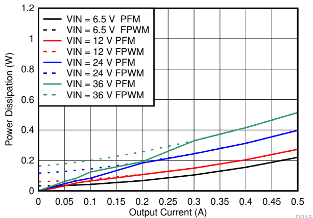
图 7-9. Power Dissipation
