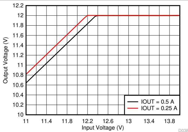
图 7-3. Dropout Voltage
