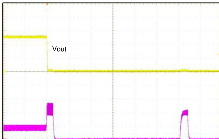
图 8-2. Hiccup Operation
