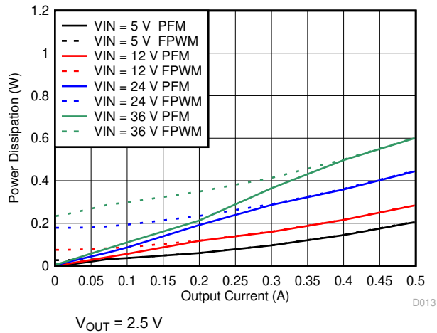
图 7-13. Power Dissipation
