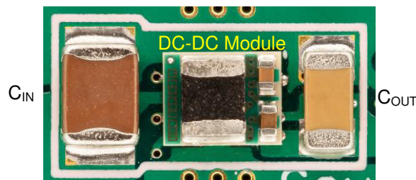
24V 至 5V、0.5A 直流/直流转换器单面布局解决方案尺寸
