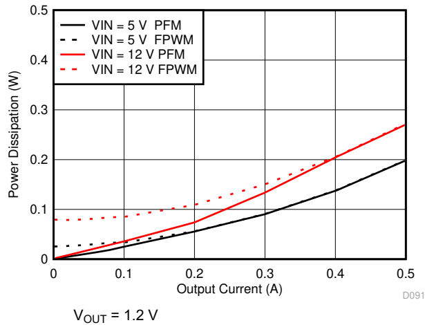
图 7-15. Power Dissipation
