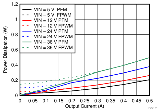
图 7-10. Power Dissipation
