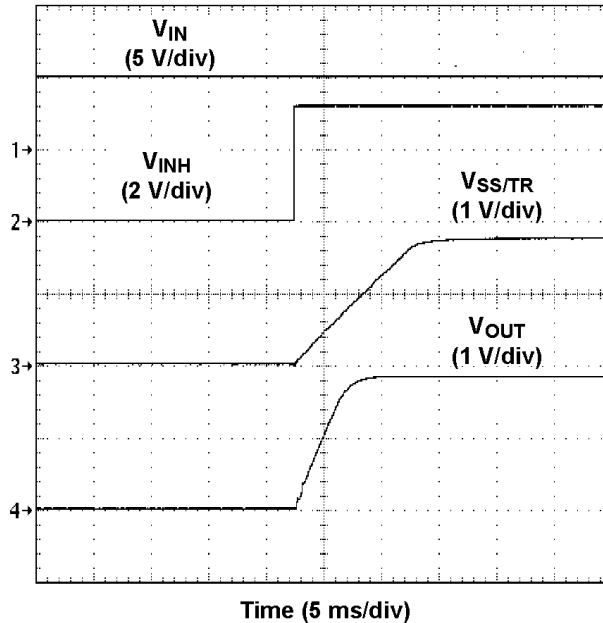
图 32. Inhibit Turn-On
