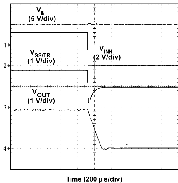
图 31. Inhibit Turn-Off
