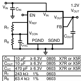
图 8-2. Schematic V_{OUT} = 1.2\text{ V}
