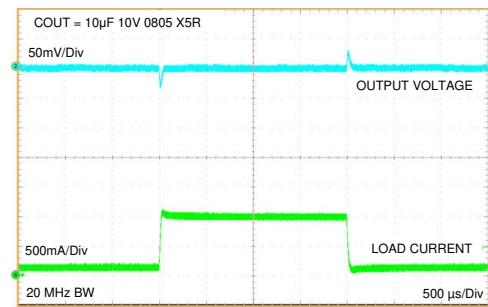
图 8-17. Load Transient V_{OUT} = 2.5\text{ V}
