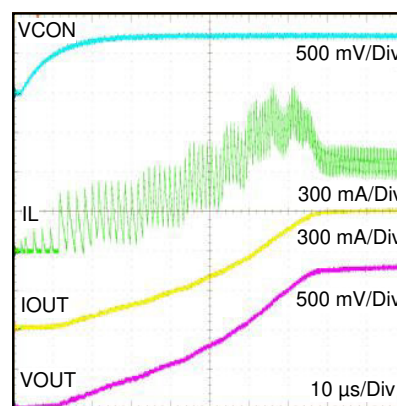
图 6-8. Startup
