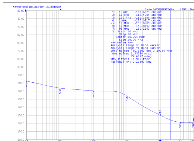
图 8-2. 测量图
