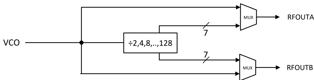
图 7-1. 通道分频器
