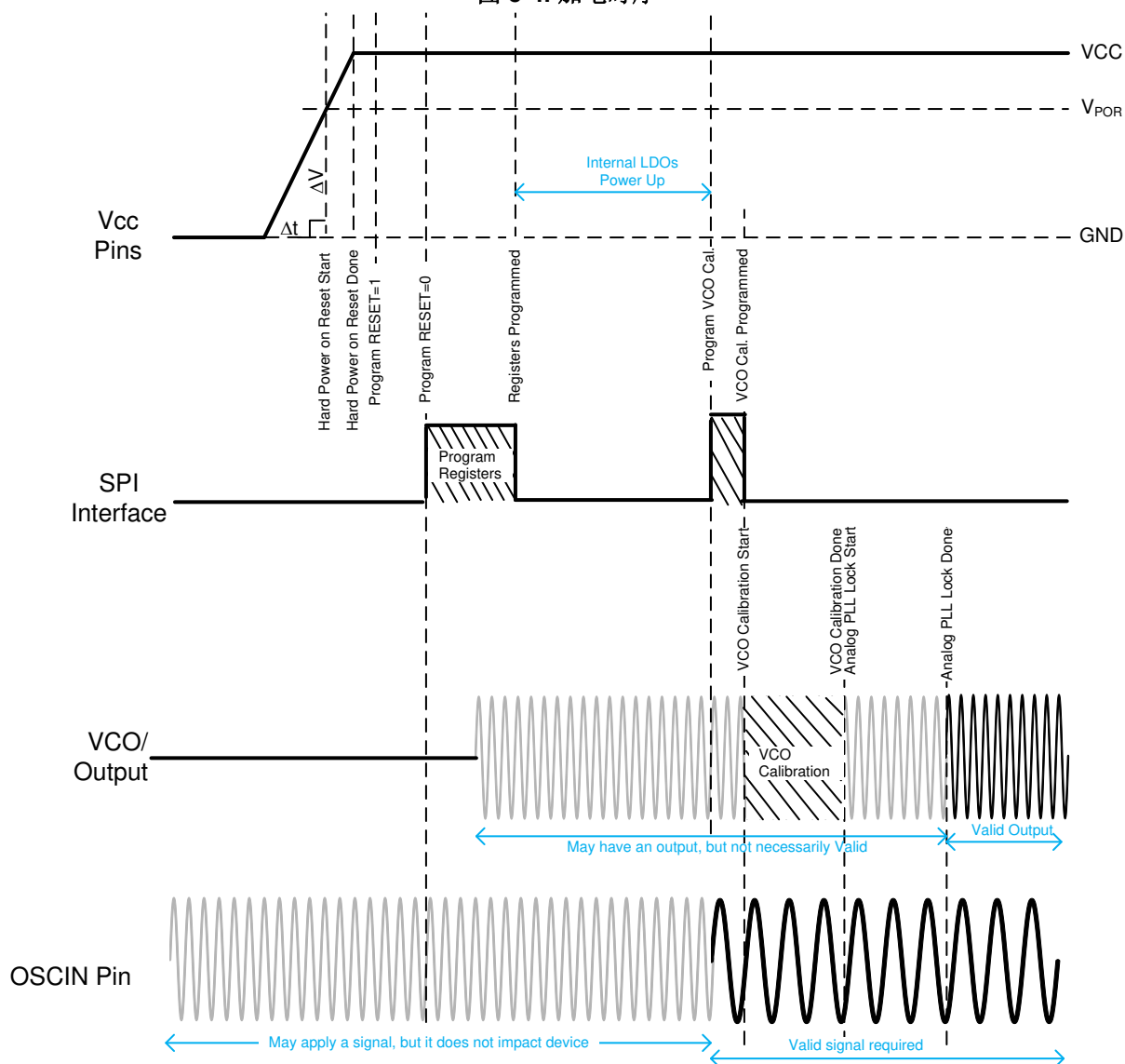
图 8-4. 加电时序
