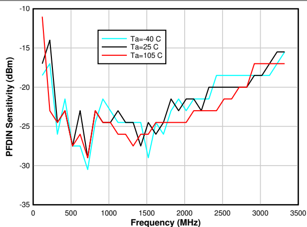
图 6-11. PFDIN 引脚输入灵敏度
