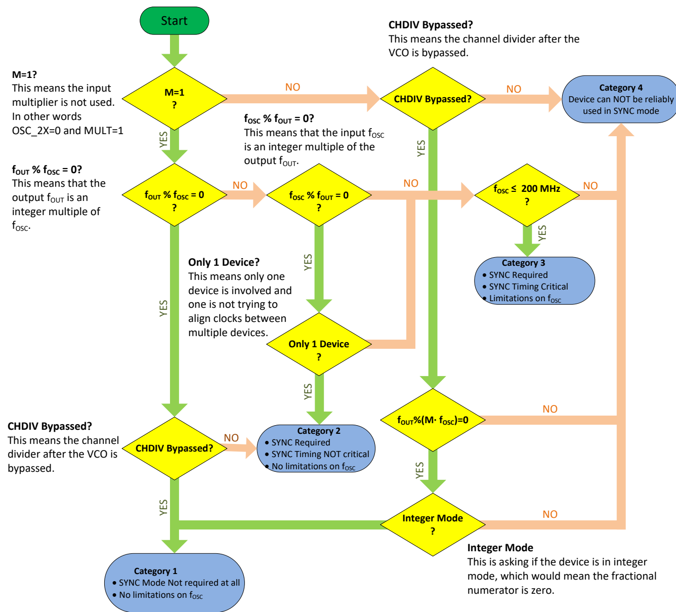
图 7-3. 同步流程图
