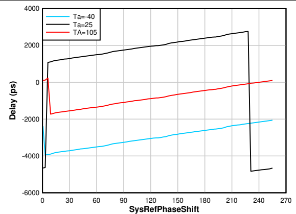
图 6-16. SysRef 延迟与温度间的关系
