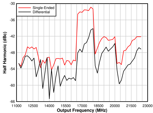
图 6-9. 启用了倍频器的输出半谐波
