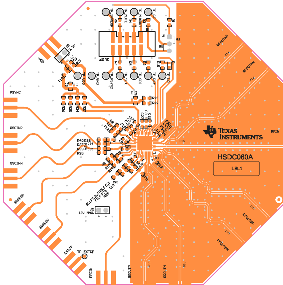
图 10-1. 布局示例
