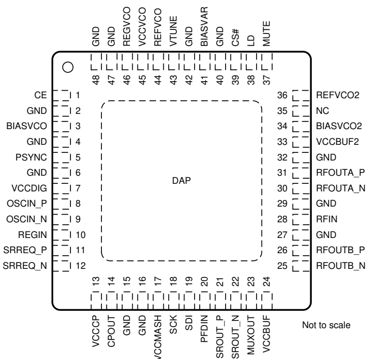
图 5-1. RTC 48 引脚 VQFN 封装 俯视图
