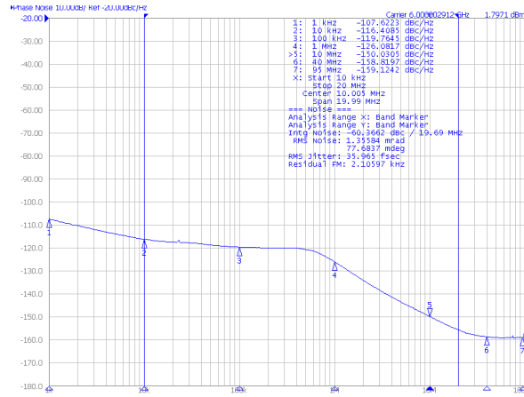
图 6-1. 闭环噪声
