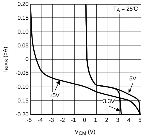
图 7. 输入偏置电流与 V_{\text{CM}} 间的关系
