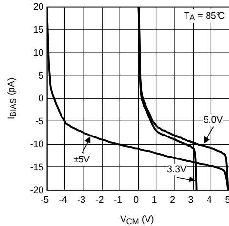
图 8. 输入偏置电流与 V_{\text{CM}} 间的关系
