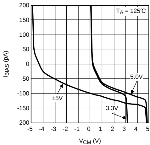
图 9. 输入偏置电流与 V_{\text{CM}} 间的关系
