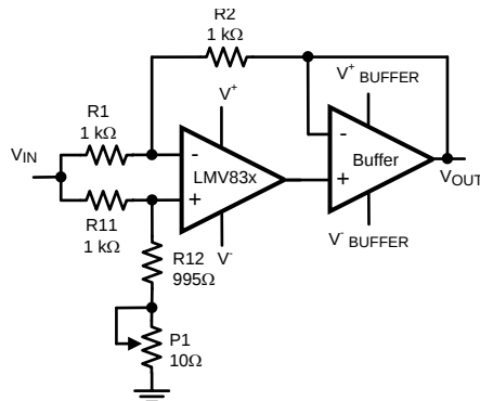
Figure 47. 交流 CMRR 测量设置
