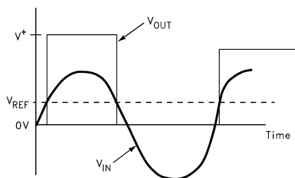
图 20. 基本比较器
