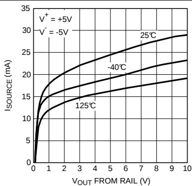
图 25. 拉电流与 V_{OUT} 间的关系
