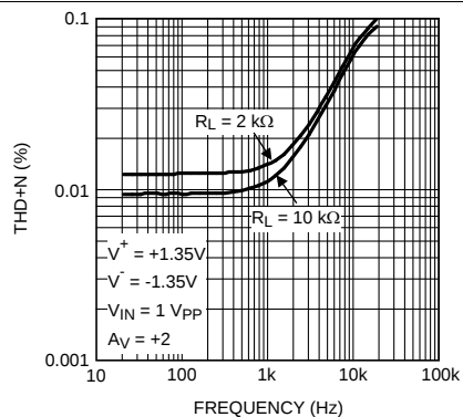
图 19. THD+N 与频率间的关系
