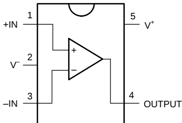
SOT-23 的 – LMV611
