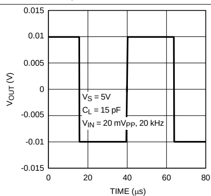
Figure 7. 小信号瞬态响应
