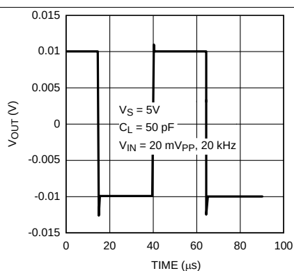
Figure 7. 小信号瞬态响应
