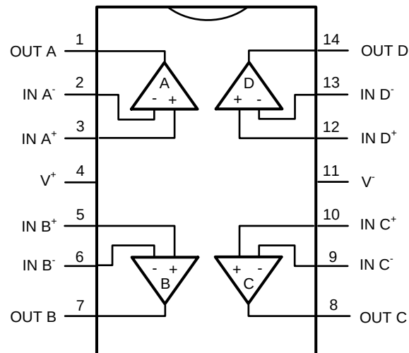
PW 封装 14 引脚 TSSOP 俯视图
