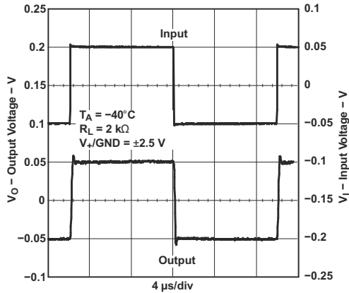
图 5-25. 小信号同相应
