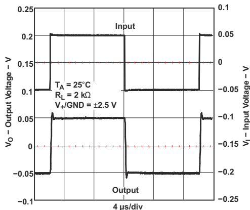
图 5-27. 小信号同相应
