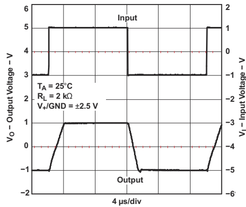
图 5-28. 大信号同相应
