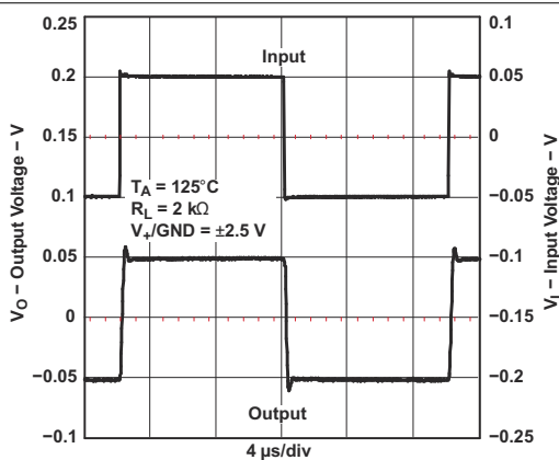
图 5-29. 小信号同相应
