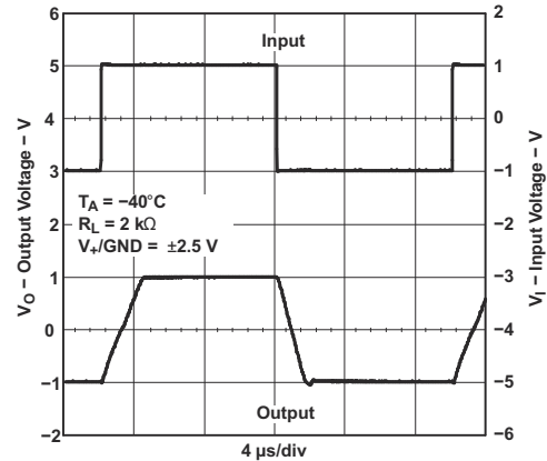
图 5-26. 大信号同相应
