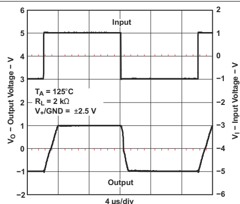
图 5-30. 大信号同相应
