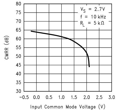
图 7-14. CMRR 与输入共模电压之间的关系
