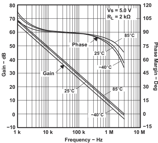
图 6-5. LMV321 频率响应与温度间的关系
