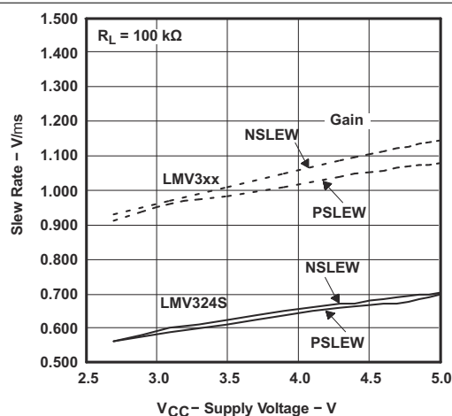
图 6-10. 压摆率与电源电压间的关系
