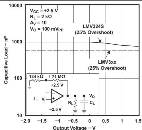
图 6-8. 稳定性与容性负载间的关系
