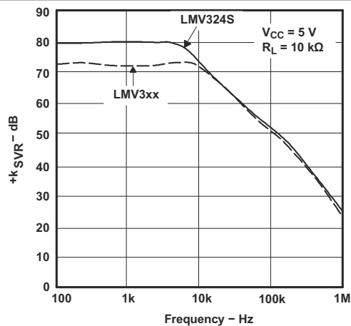
图 6-20. +k_{SVR} 与频率间的关系
