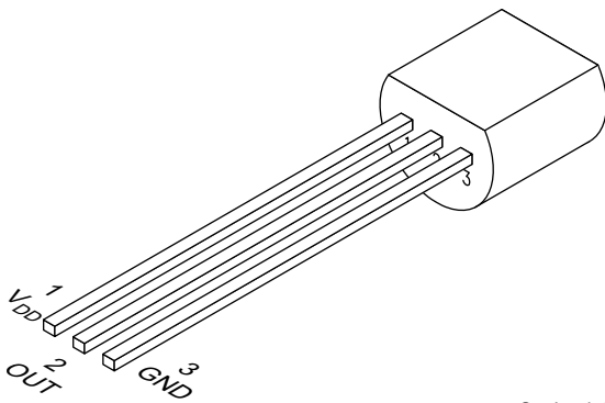
图 5-3. LP 封装 3 引脚 TO-92 (顶视图)
