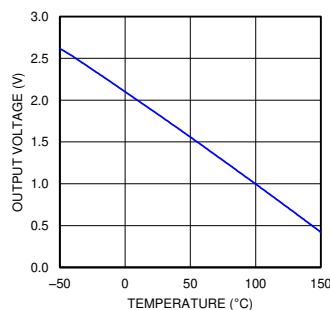
图 8-2. 模拟输出传递函数
