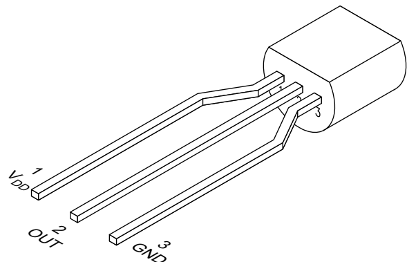
图 5-4. LPM 封装 3 引脚 TO-92 (顶视图)
