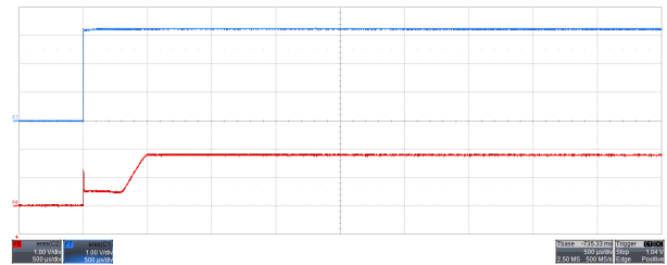
图 8-5. 输出导通响应时间：带 1.1nF 容性负载， V_{\text{DD}} = 3.3\text{V}
