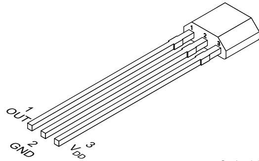
图 5-2. LPG 封装 3 引脚 TO-92S (顶视图)
