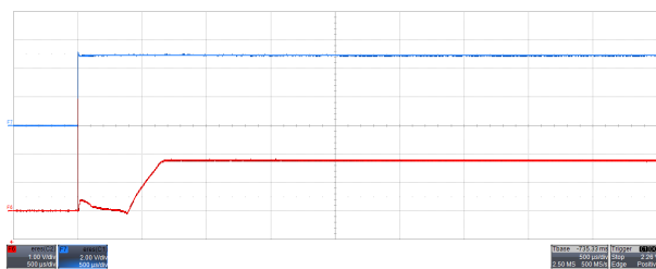
图 8-4. 输出导通响应时间：无容性负载， V_{\text{DD}} = 3.3\text{V}
