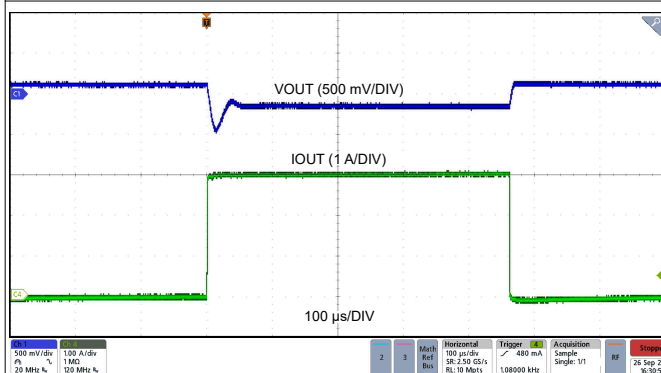
LMR66430R5R V_{OUT} = 5V 400kHz (自动) 0A 至 3A, 1A/ \mu s 修复
