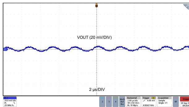
图 8-10. 输出电压纹波
