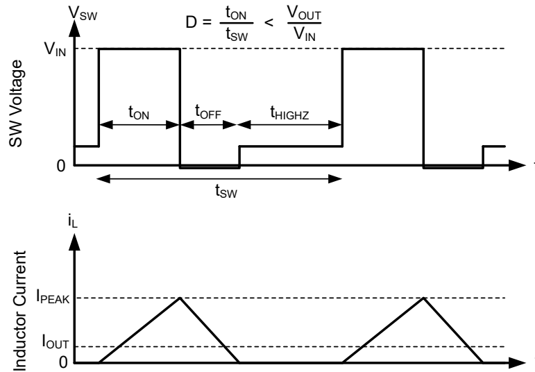
图 7-17. PFM 运行
