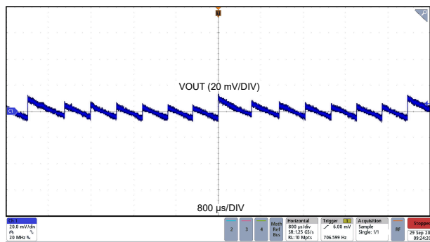
图 8-11. 输出电压纹波
