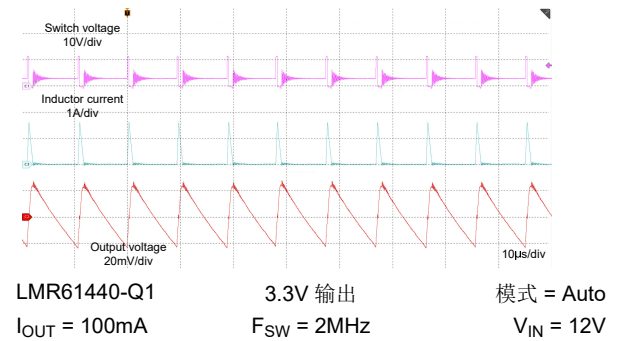
图 8-11. 稳态波形
