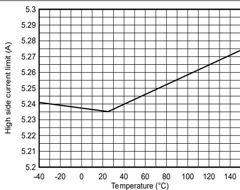
图 6-1. 高侧 MOSFET 电流限制
