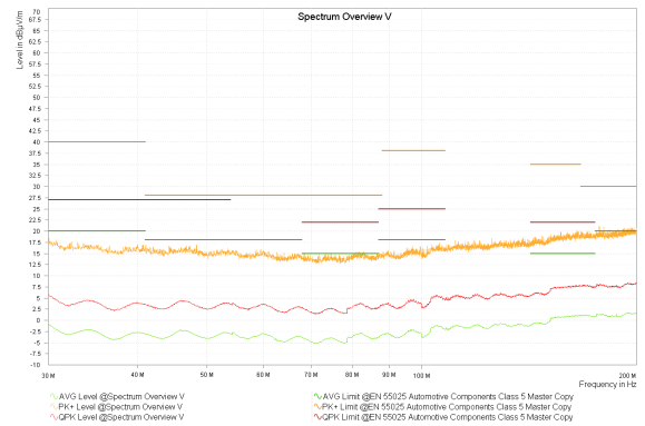
图 8-15. 辐射 EMI (单极) 与 CISPR 25 限值对比
