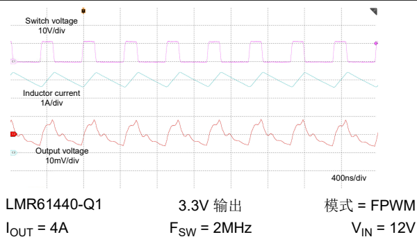
图 8-12. 稳态波形
