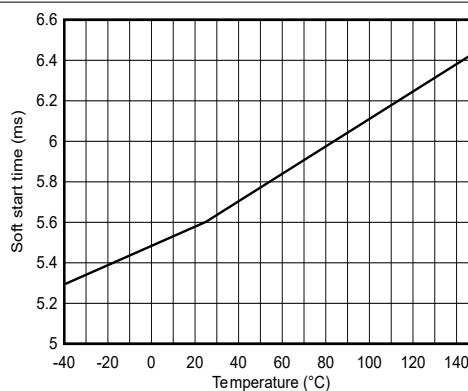
图 6-6. 软启动时间
