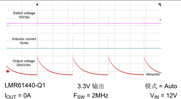
图 8-13. 稳态波形
