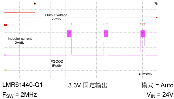
图 8-10. 应用短路
