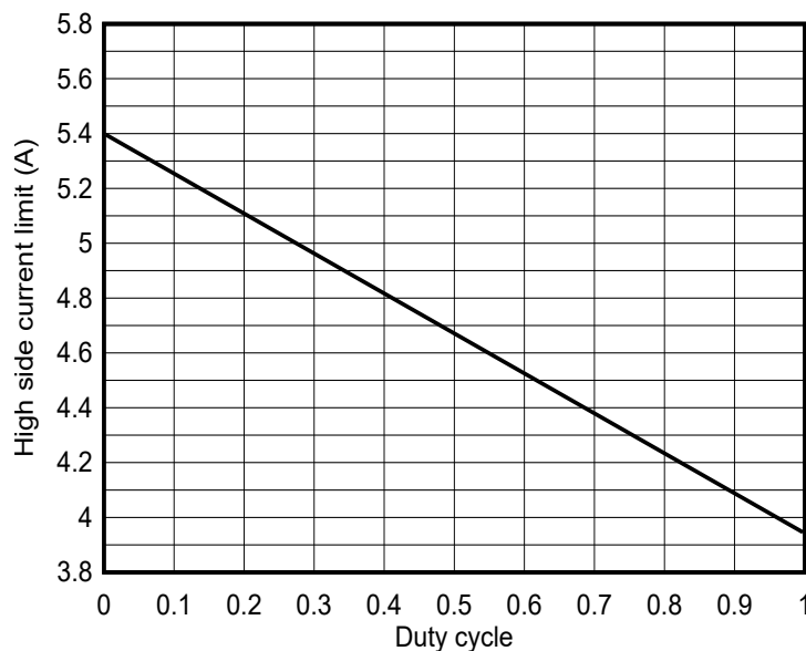
图 7-4. 典型高侧电流限制 I_{HS-LIM} 与占空比 D 的函数关系
