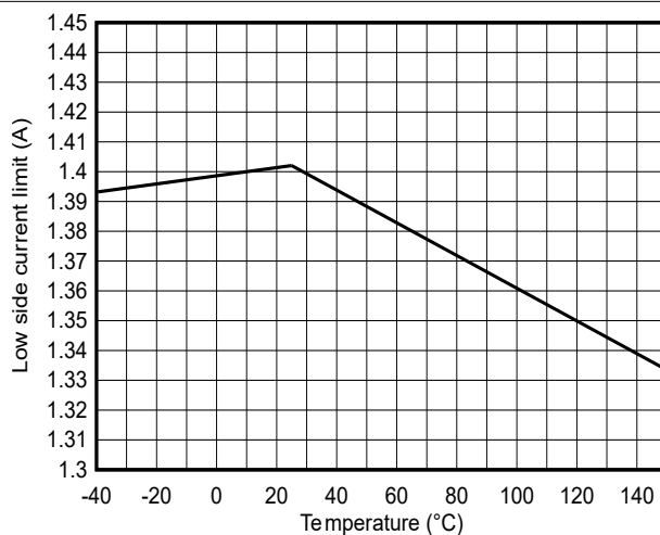
图 6-2. 低侧 MOSFET 电流限制
