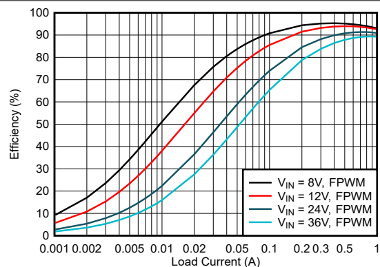
器件类型 = 1A 5V 输出 模式 = FPWM F_{sw} = 400kHz
