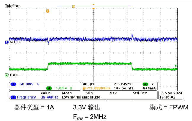
图 8-21. 0.5A 至 1A 负载瞬态
