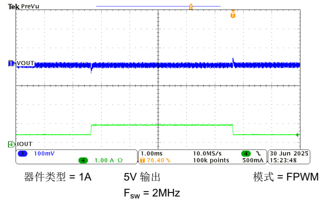
图 8-19. 0.5A 至 1A 负载瞬态
