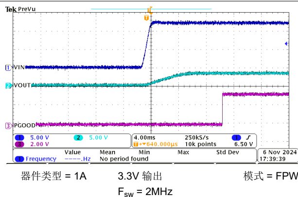
图 8-16. 启动
