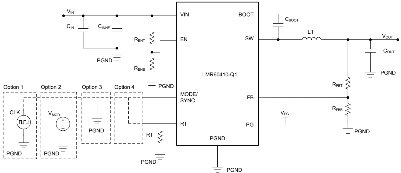
图 8-1. LMR60410-Q1 参考原理图
