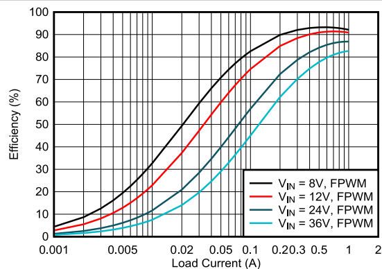
器件类型 = 1A 5V 输出 模式 = FPWM F_{sw} = 2MHz
