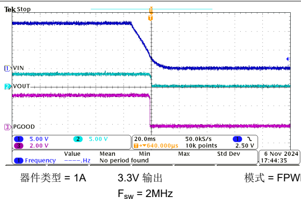
图 8-17. 关断
