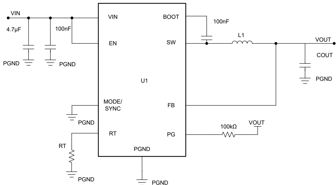
图 8-34. 应用电路示例
