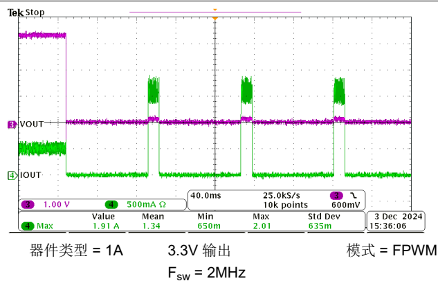
图 8-22. 应用短路
