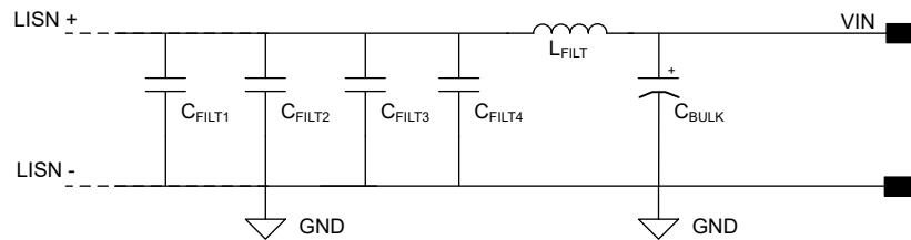
图 8-33. 典型输入 EMI 滤波器原理图
