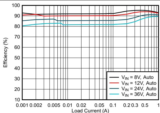
器件类型 = 1A 5V 输出 模式 = AUTO F_{sw} = 400kHz
