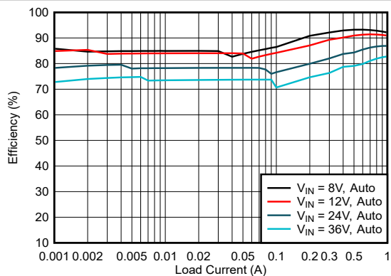
器件类型 = 1A 5V 输出 模式 = AUTO F_{sw} = 2MHz
