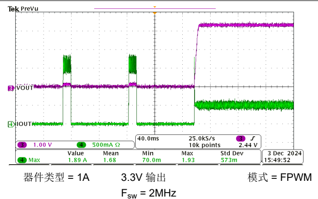
图 8-23. 短路恢复
