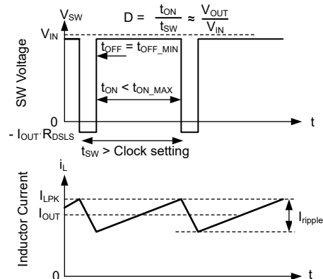
图 7-10. 压降波形
