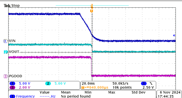
图 8-4. 压降电压
