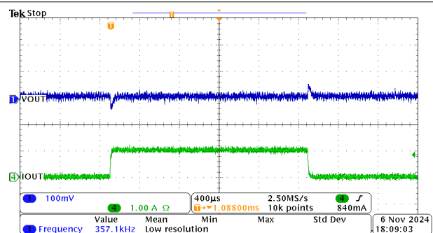
图 8-7. 0A 至 1A 负载瞬态
