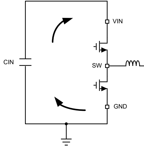
图 8-12. 具有快速瞬变的电流环路
