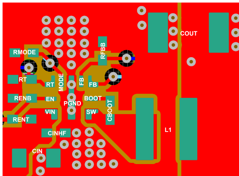
图 8-13. 示例布局
