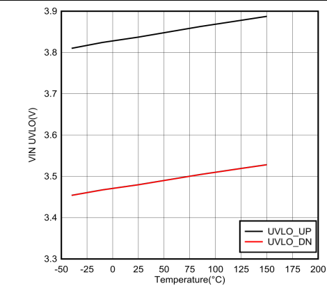
图 6-11. V_{IN} UVLO Versus Temperature
