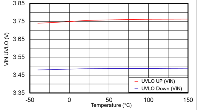
图 6-10. V_{IN} UVLO
