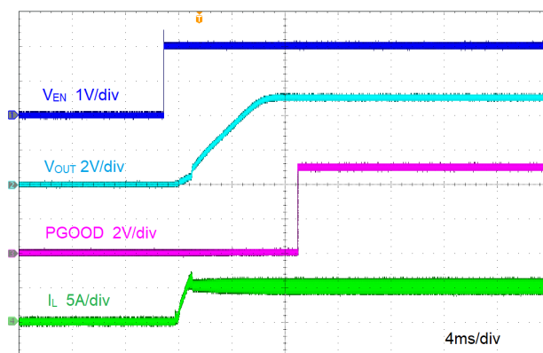
图 8-5. 由 EN 启动
