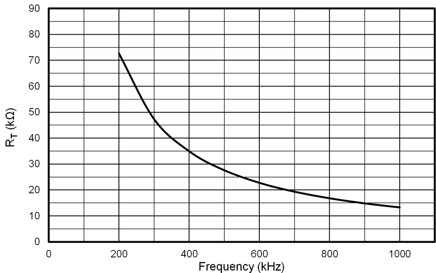
图 7-4. R_T 与频率曲线间的关系
