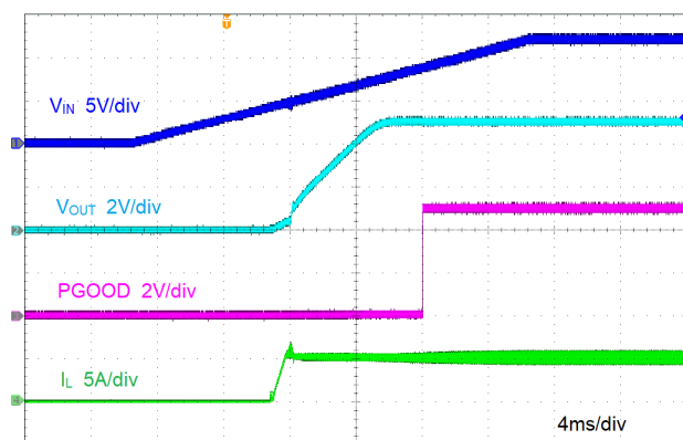
图 8-4. 由 V_{IN} 启动
