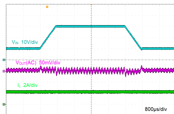
图 8-7. 线路瞬态
