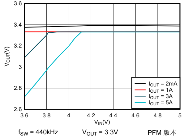
图 6-8. 3.3V 压降
