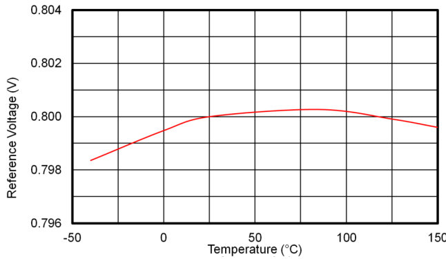
图 6-11. 基准电压
