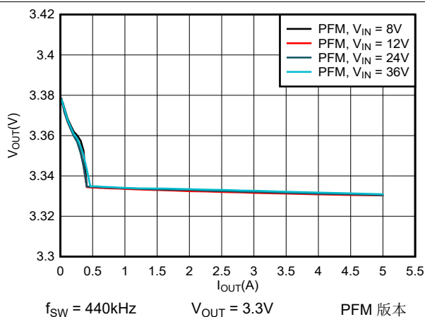
图 6-5. 3.3V 负载调整
