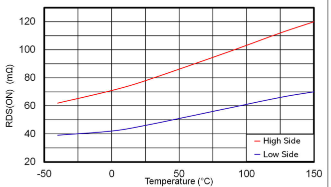
图 6-12. 高侧和低侧开关 R_{DS(on)}
