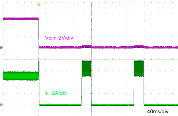
图 8-8. 短路保护
