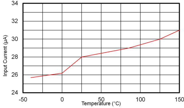
图 6-9. 非开关输入电源电流
