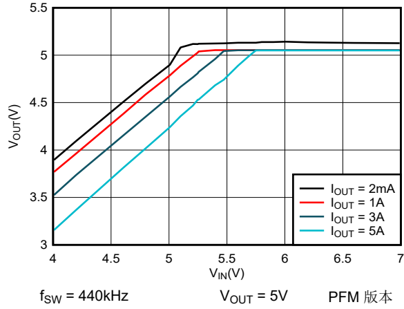
图 6-7. 5V 压降
