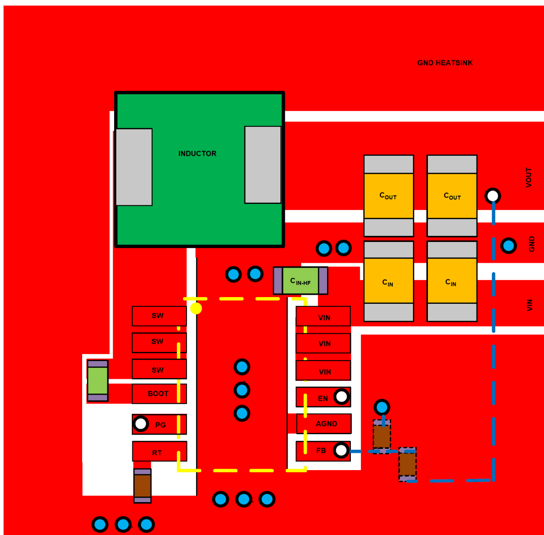
图 8-10. 布局
