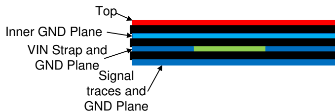
图 11-2. Example Layout
