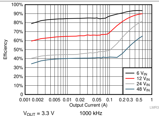
图 22. Efficiency
