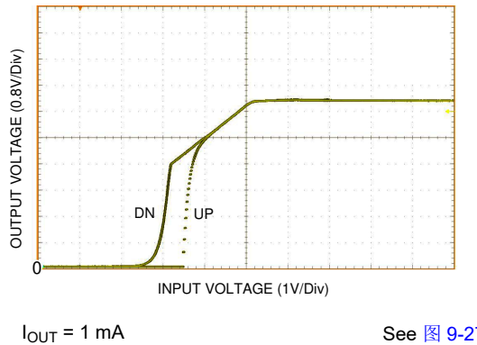
图 7-5. UVLO Thresholds
