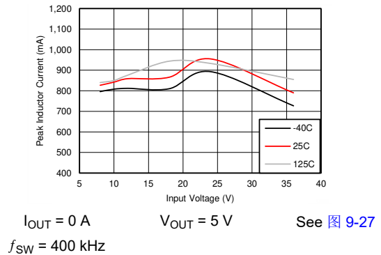
图 7-6. I_{PEAK-MIN}
