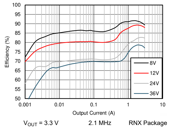
图 9-8. Efficiency
