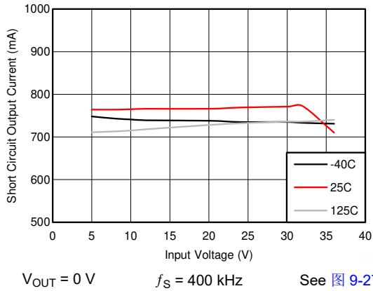
图 7-3. Short-Circuit Output Current
