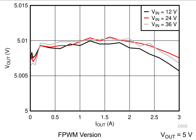
图 7-6. Load Regulation
